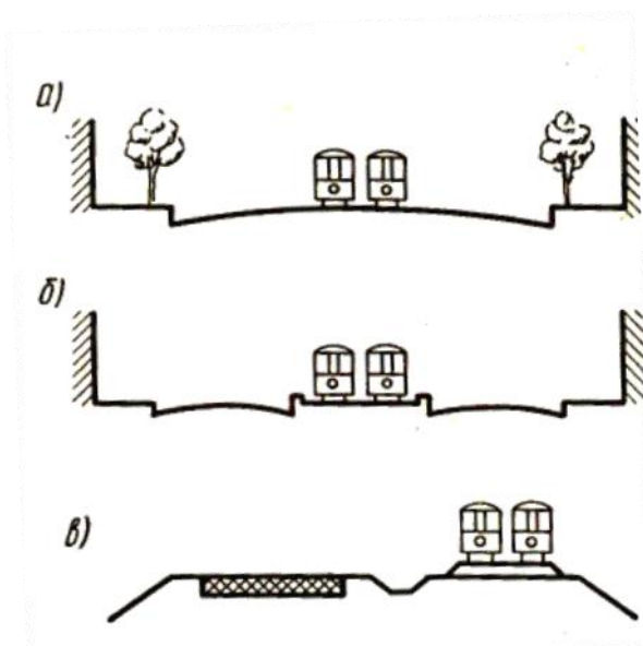
Рисунок 1.4 – Типи трамвайного полотна
