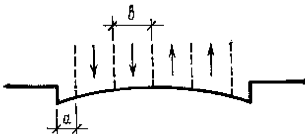
Рисунок 1.2 – Схема для розрахунку ширини проїзної частини
