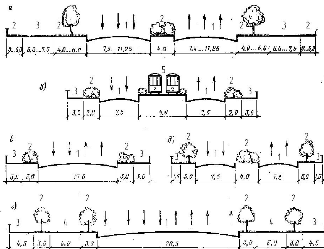
Рисунок 1.1 – Поперечні профілі магістральних вулиць 1 – проїзна частина; 2 – розділювальні смуги та смуги озеленення; 3 – тротуар; 4 – бічні проїзди; 5 – трамвайне полотно на центральній розділювальній смузі
