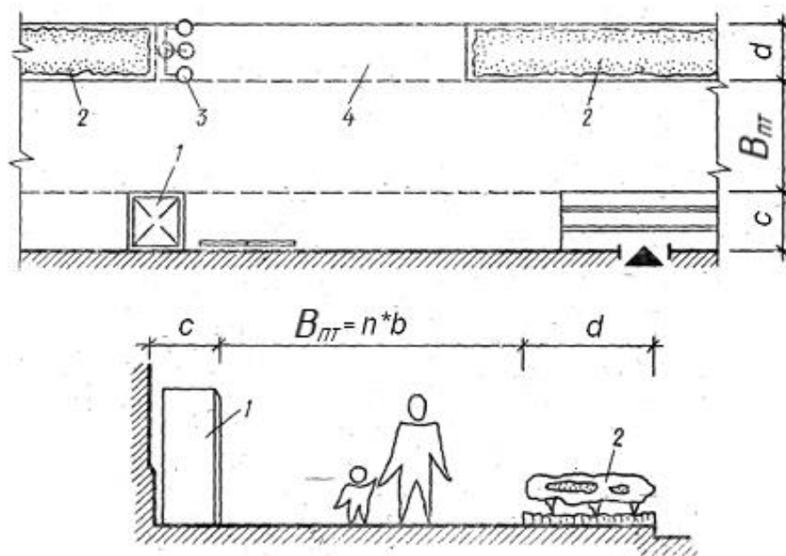
Рисунок 1.3 – Планувальна схема тротуару
