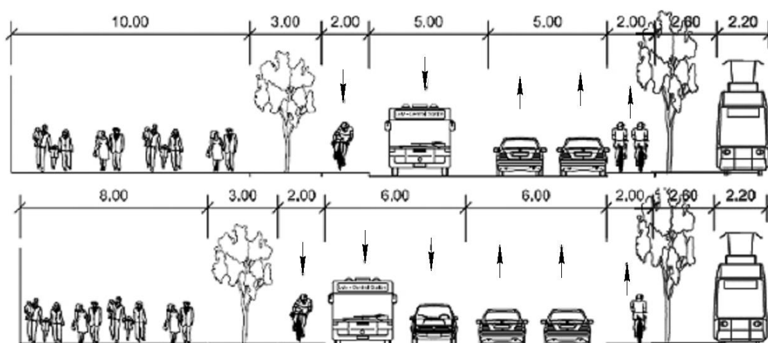
Рисунок 3.1 – Приклад оформлення поперечного профілю міської магістральної вулиці
