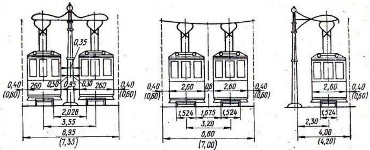
Рисунок 1.5 – Габаритні розміри трамвайного полотна ( у дужках зазначені розміри для проектування ліній швидкісного трамвая)
