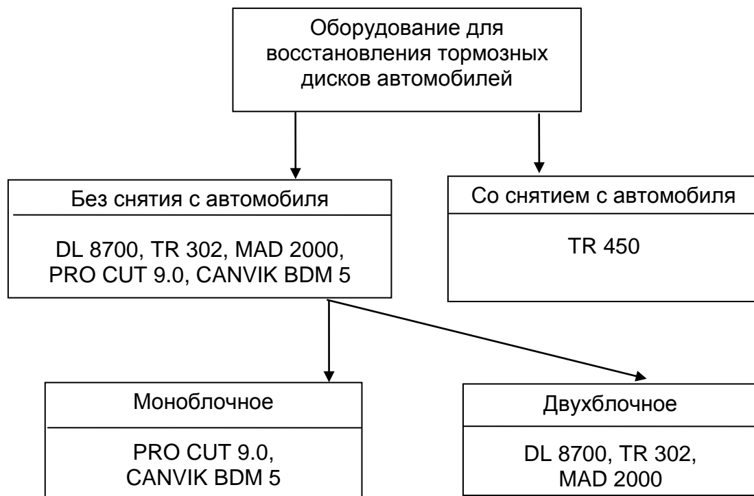
Рис. 1. - Оборудование для восстановления тормозных дисков автомобилей
