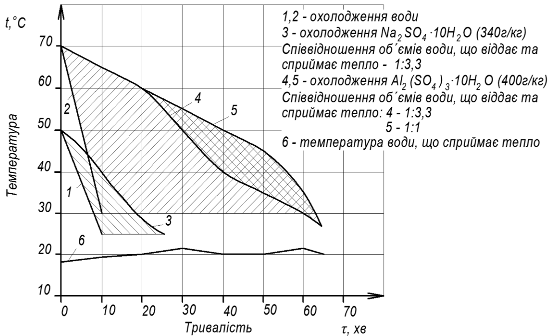
Рис. 3 Сравнительная характеристика аккумуляирования тепла сульфатом алюминия ( \text{Al}_2(\text{SO}_4)_3 \cdot 18\text{H}_2\text{O} ) и сульфатом натрия ( \text{Na}_2\text{SO}_4 \cdot 10\text{H}_2\text{O} )
