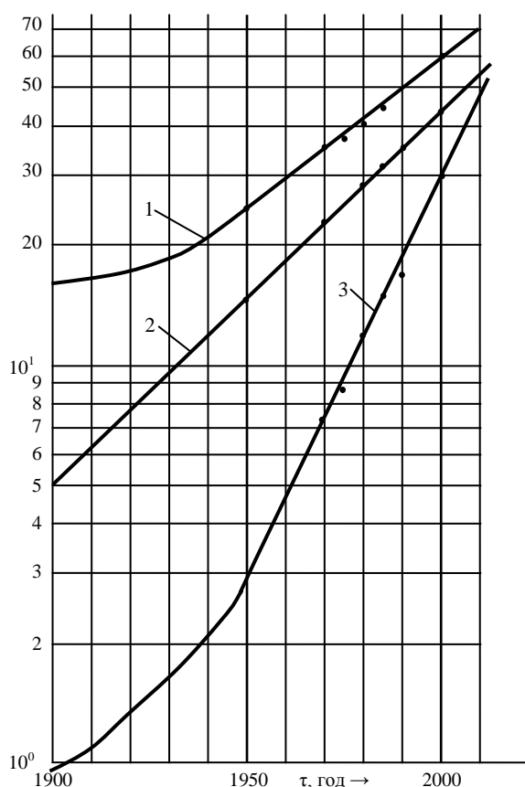
Рис.1 Изменение численности населения Земли, потребления энергоресурсов и удельного энергопотребления 1 – народонаселение, млрд. человек · 10 -1 ; 2 – удельное энергопотребление, т. у. т · 10 -1 /
