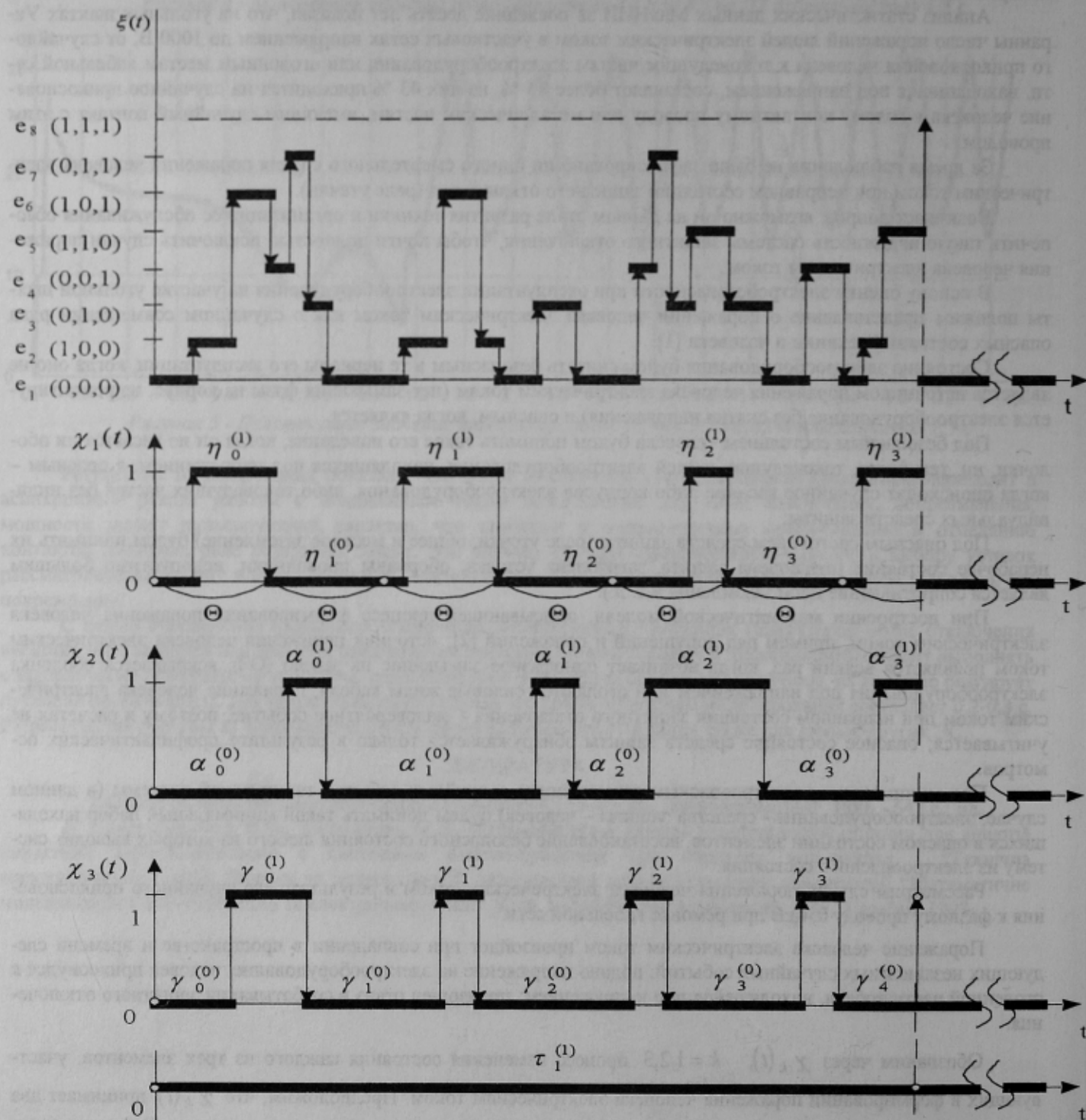
Рисунок 1 - Возможная реализация марковского процесса
