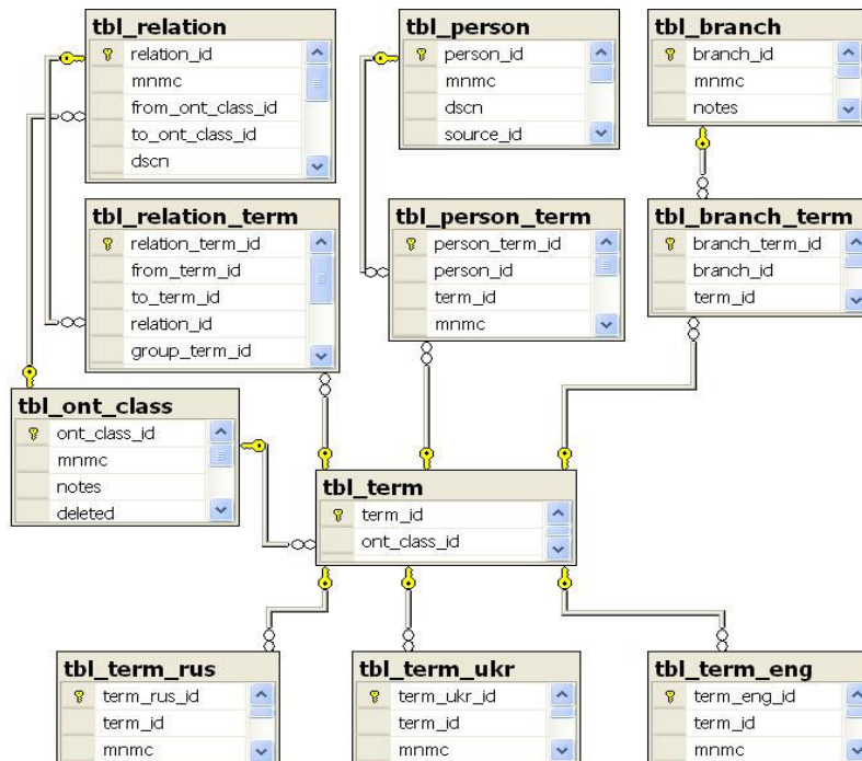
Рисунок 3 – Общая схема лексикографической базы данных
