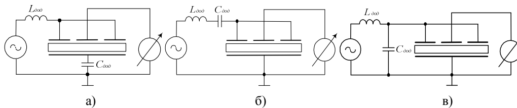
Рисунок 3 – Перетворювач ЗП-19 з додатковими індуктивністю і ємністю
