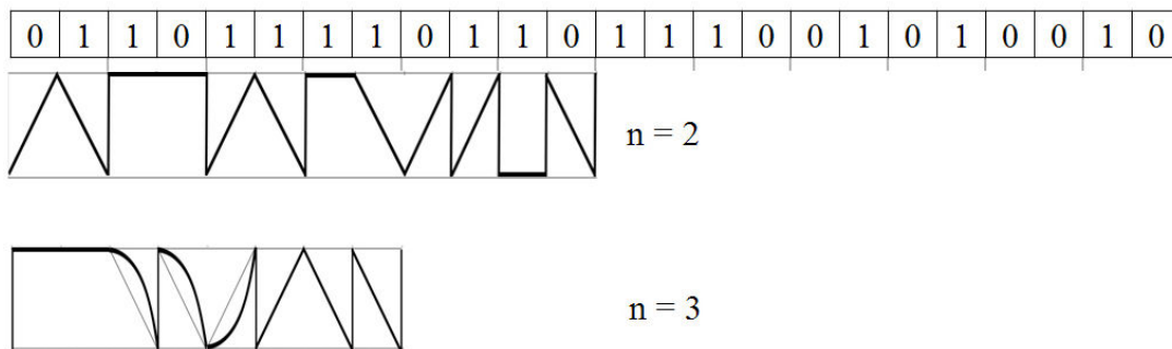
Рис.1. Приклади заміщення n – бітових послідовностей сигнальними послідовностями.
