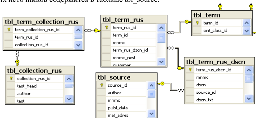
Рисунок 4 – Группа таблиц русского языка
