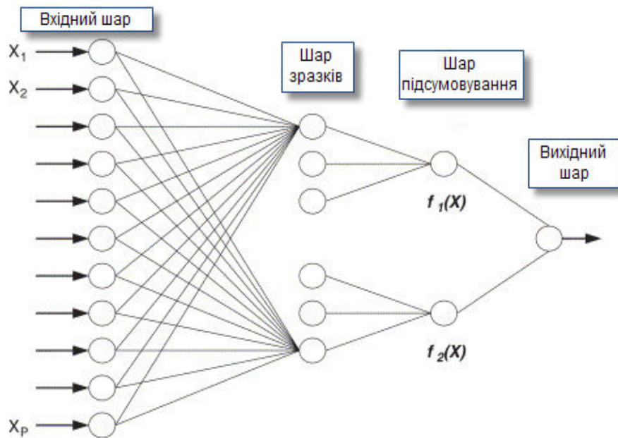
Рисунок 3 – Архітектура PNN
