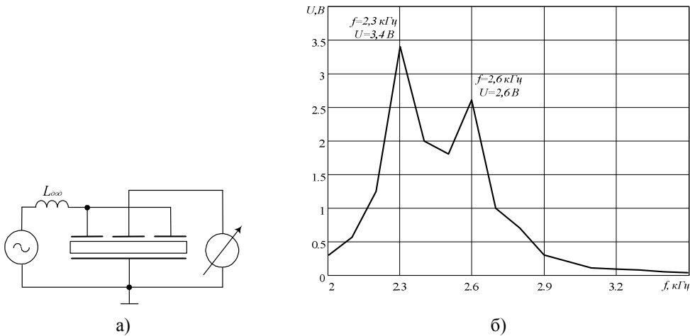
Рисунок 2 – Вимірювальна схема (а) та АЧХ п'єзоперетворювача ЗП-19 (б) при L_{000} = 325 мГн
