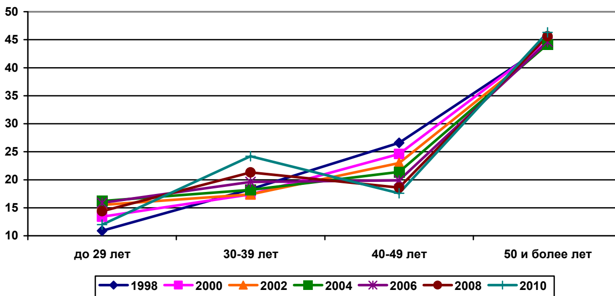
Рис.2а. Динамика возрастной структуры ППС, %
