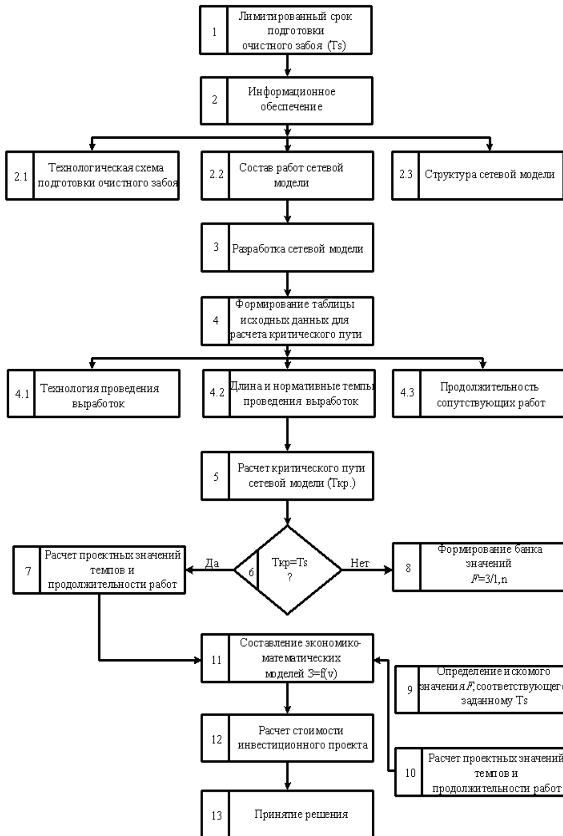
Рис. 3. Алгоритм оптимизации сетевой модели воспроизводства фронта очистных работ угольной шахты
