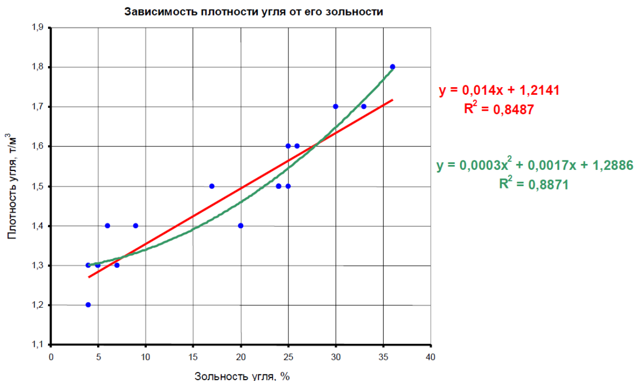
Рисунок 1 – Вид регрессионной зависимости, построенной с помощью Excel
