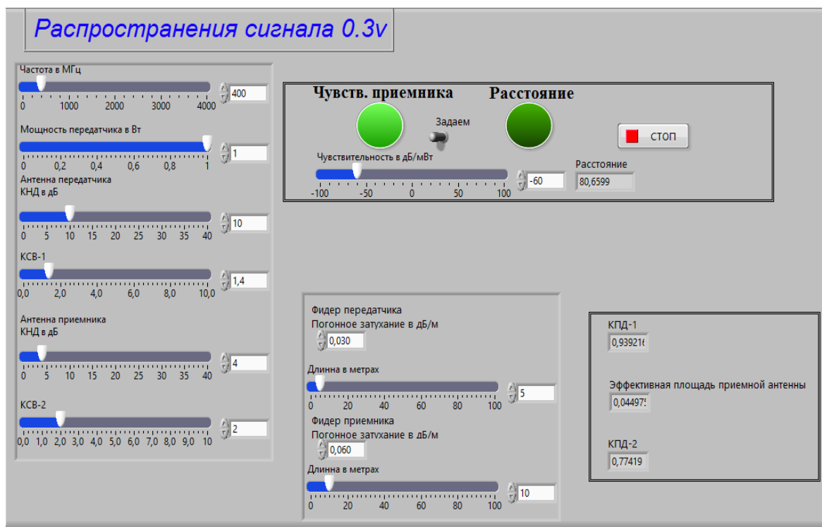
Рисунок 2 – Лицевая панель модели LabView распространения радиоволн
