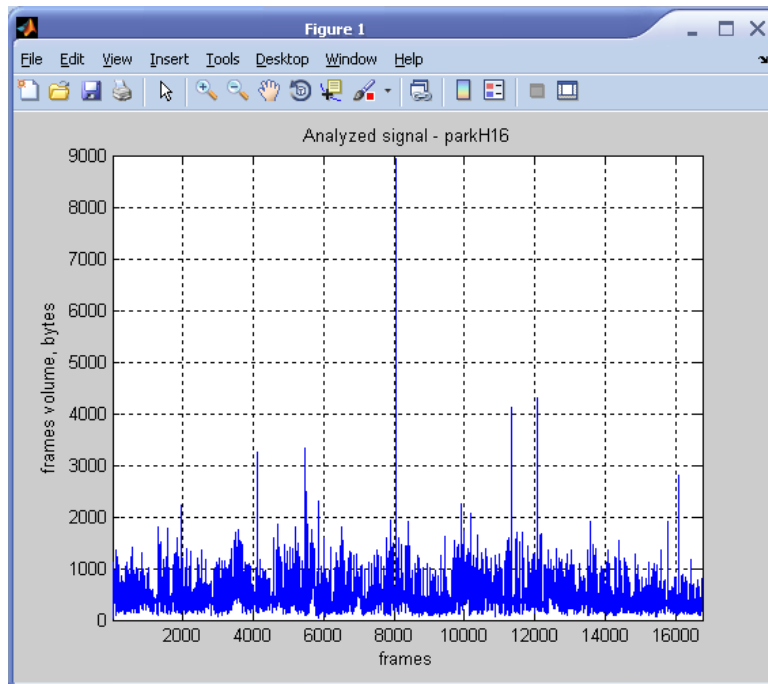
Рисунок 1 – Временной ряд parkH16
