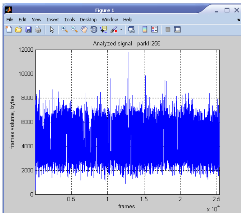
Рисунок 3 – Временной ряд parkH256
