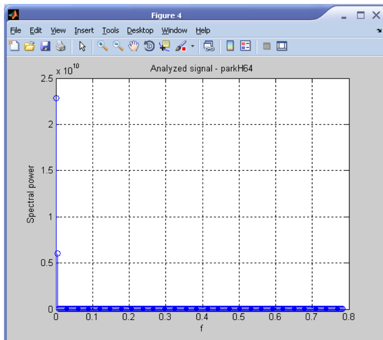
Рисунок 14 – Спектральная плотность временного ряда parkH64
