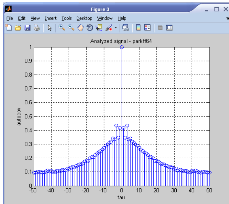
Рисунок 10 – АКФ временного ряда parkH64
