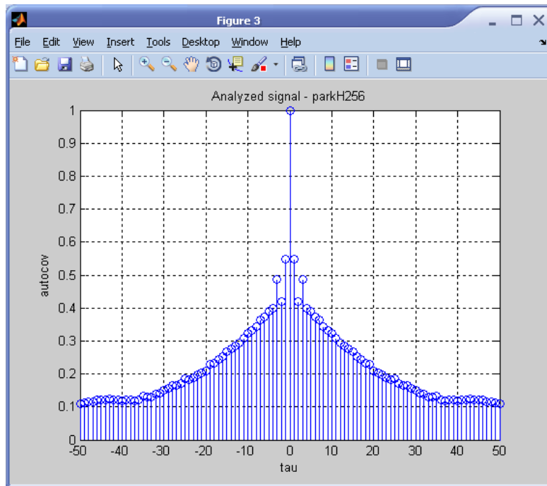
Рисунок 11 – АКФ временного ряда parkH256
