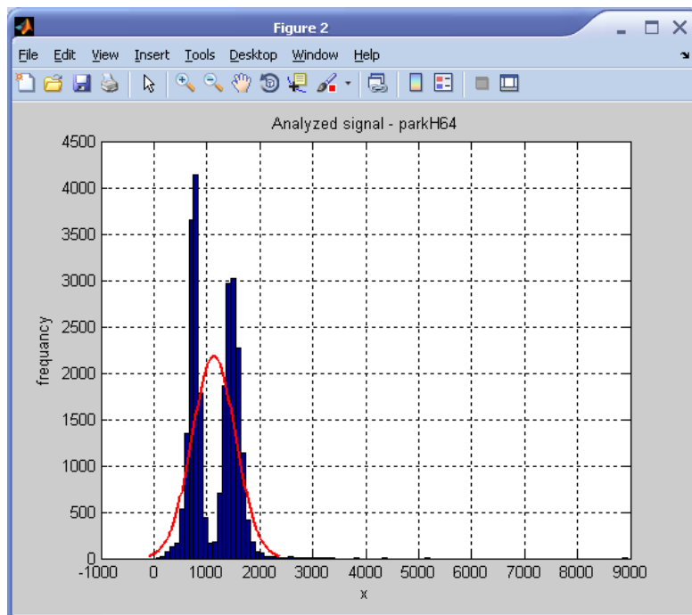
Рисунок 6 – Плотность распределения временного ряда parkH64
