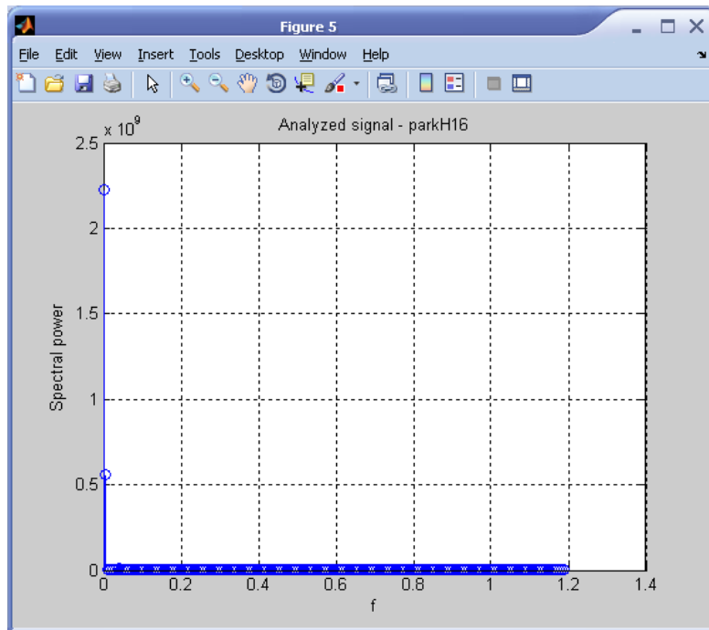
Рисунок 13 – Спектральная плотность временного ряда parkH16
