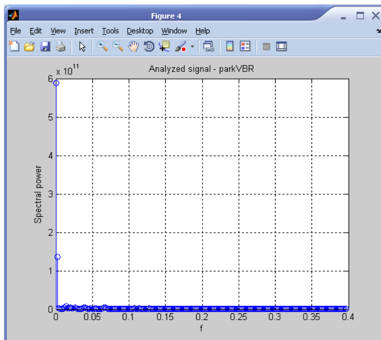
Рисунок 16 – Спектральная плотность временного ряда parkVBR
