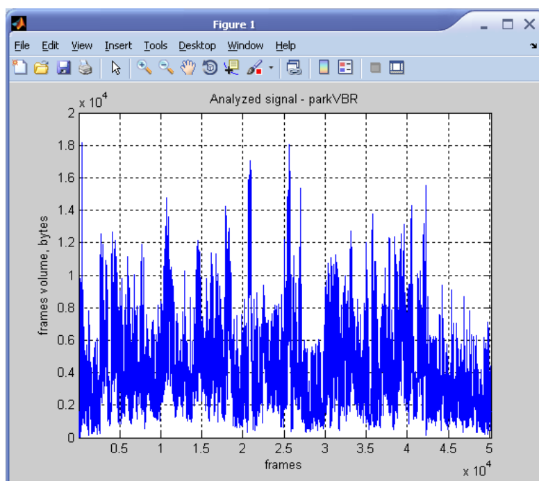
Рисунок 4 – Временной ряд parkVBR
