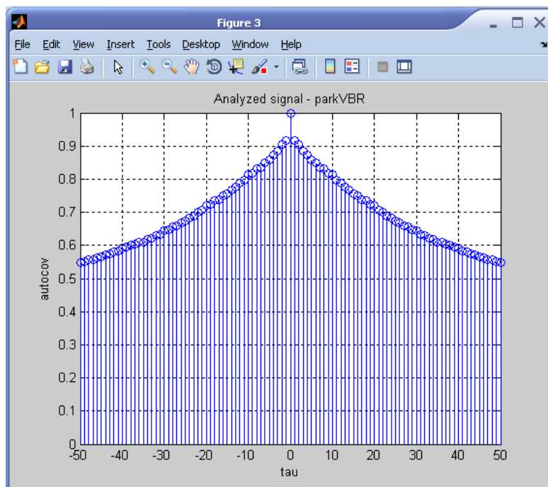
Рисунок 12 – АКФ временного ряда parkVBR
