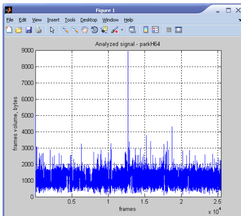
Рисунок 2 – Временной ряд parkH64
