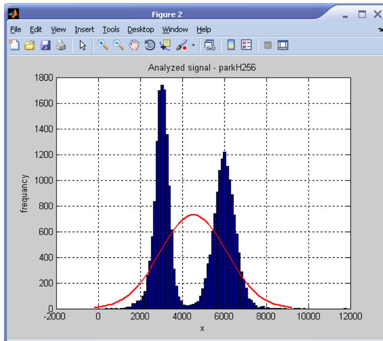
Рисунок 7 – Плотность распределения временного ряда parkH256
