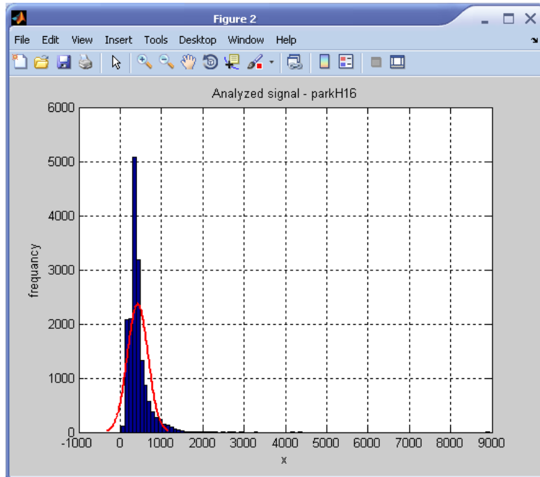
Рисунок 5 – Плотность распределения временного ряда parkH16
