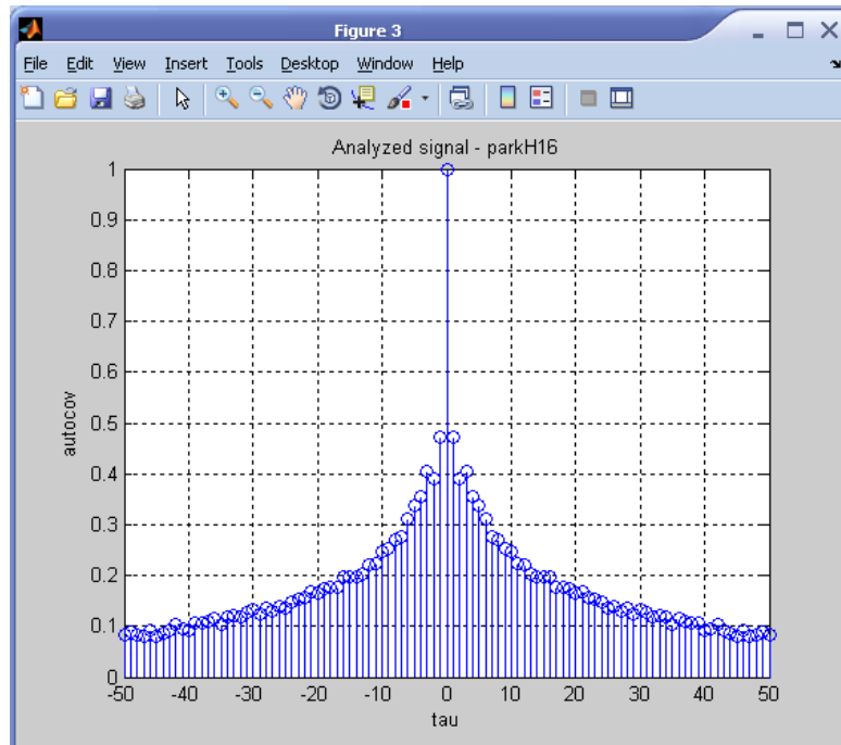
Рисунок 9 – АКФ временного ряда parkH16
