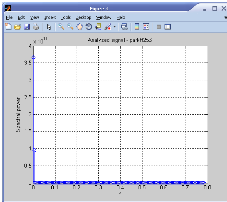
Рисунок 15 – Спектральная плотность временного ряда parkH256
