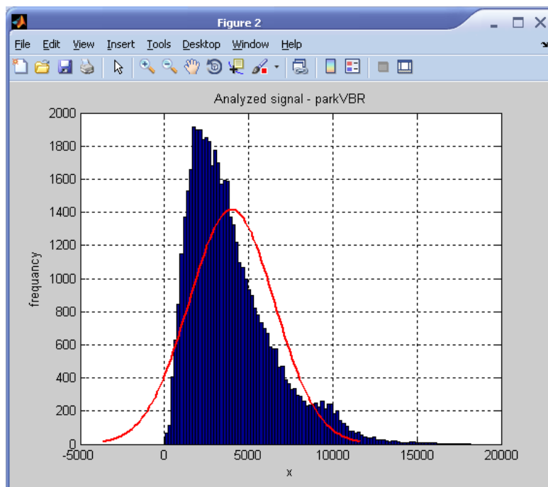
Рисунок 8 – Плотность распределения временного ряда parkVBR
