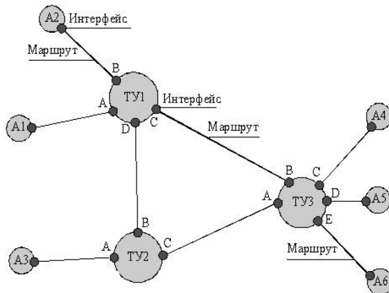
Рис. 1.1. Телекоммуникационная сеть
