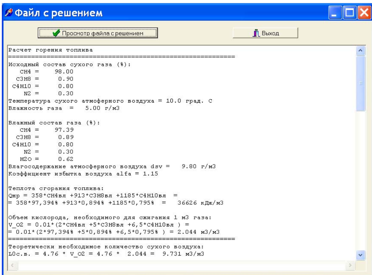
Рис.9 – Вивід у вікно вмісту файлу «решення.txt»
