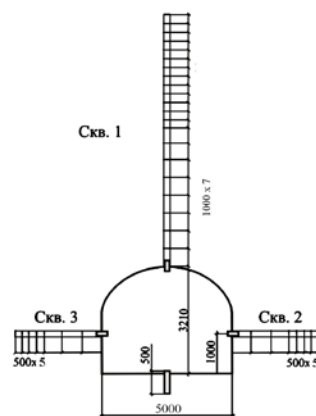
Рис. 2 – Схема замерной станции
