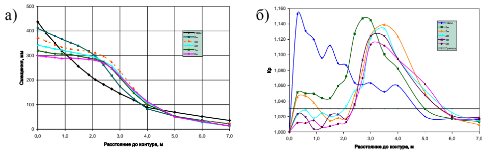
Рис. 3 – Смещения глубинных реперов в кровле выработки с рамно-анкерной крепью (а) и изменения коэффициента разрыхления на участках скважины между глубинными реперами (б) в зависимости от времени установки анкерной крепи после выемки породы в забое на 20,60,100,200 и 300 сутки наблюдений
