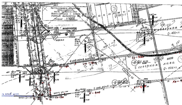
Рис. 1 – Выкопировка из плана горных выработок по пласту m_4^0
