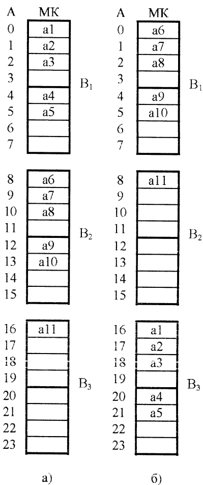
Рисунок 3 – Варианты размещения, эквивалентные в силу эвристики 1
