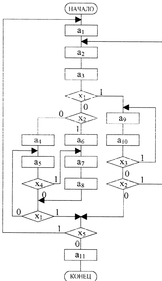
Рисунок 1 – Граф-схема алгоритма G
