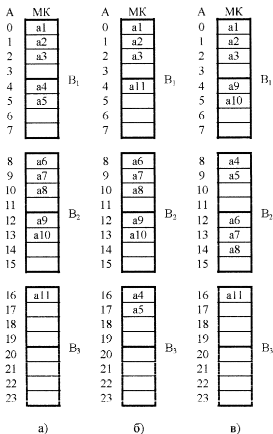
Рисунок 2 – Примеры вариантов размещения микрокоманд в управляющей памяти
