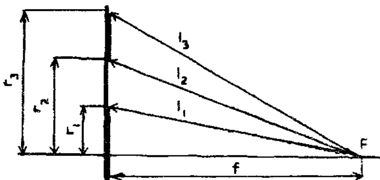
Рисунок 1 – Определение фокусного расстояния зональной антенны
