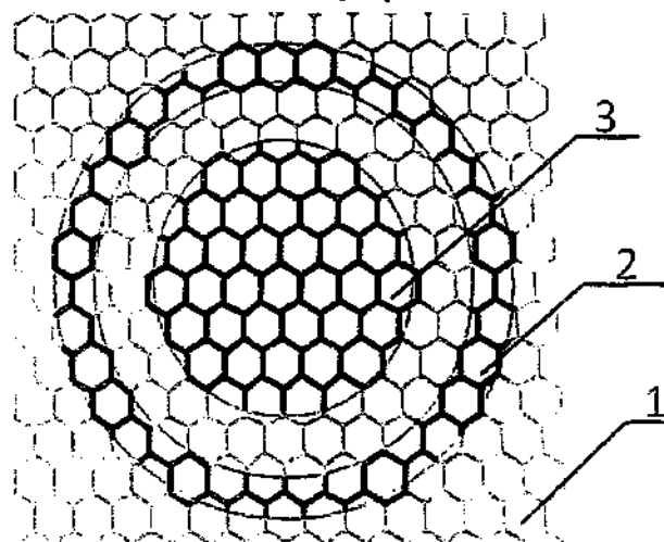
Рисунок 2 – Схематическое изображение складного антенного отражателя (1 - радиопрозрачное основание, 2 – кольцевая концентрическая поверхность, 3 - центральный диск)
