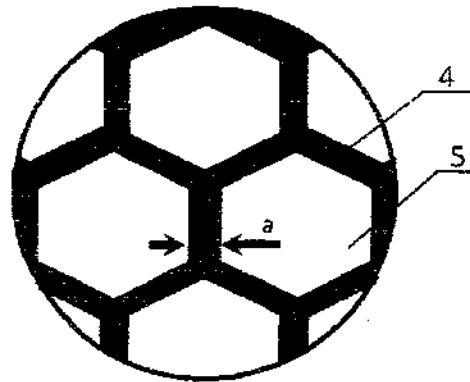
Рисунок 3 – Сотовая конструкция в увеличенном виде 4 – соединительная поверхность, 5 – сота
