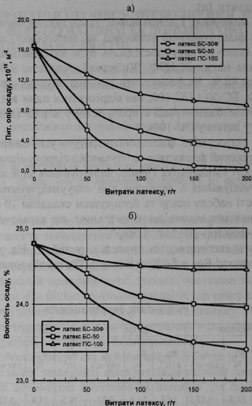
Рис. 1 Вплив витрат латексних флокулянтів на: а – питомий опір осаду; б – вологість осаду.
