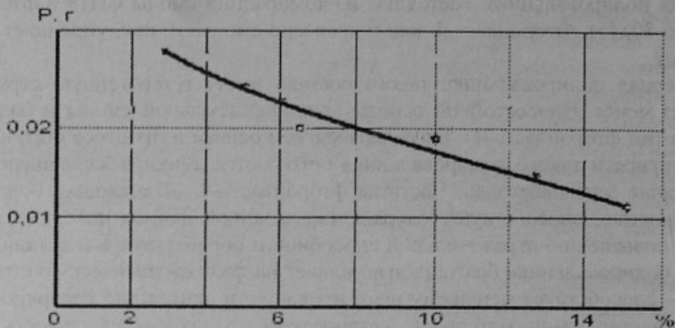
Рис.2. Залежність износу полірувальника від вмісту абразивного порошку фторопласта-4
