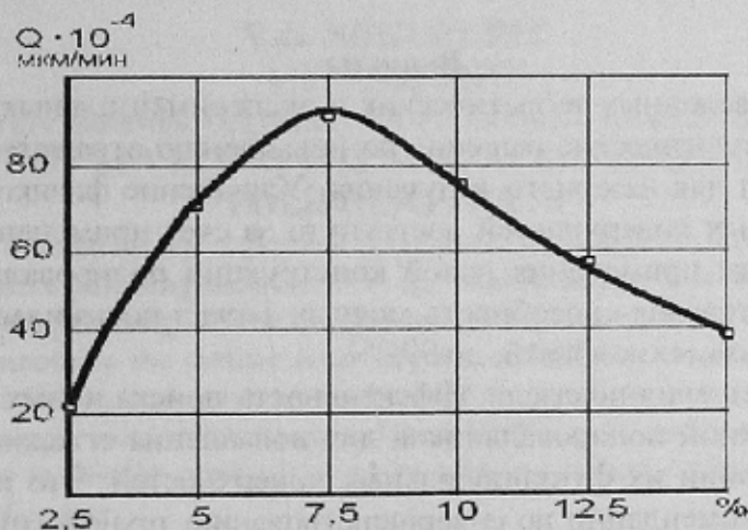
Рис.1. Зависимость съема меди марки Моб от содержания износостойкого высокодисперсного порошка фторопласта 4 в композиционном составе полировальника
