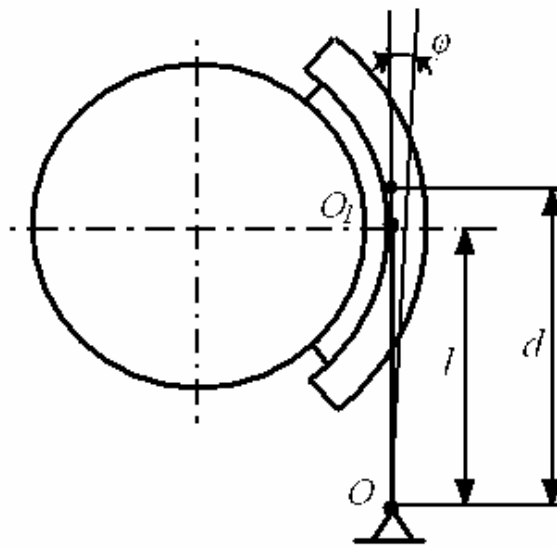
Рисунок 1 – Розрахункова схема оберту балки
