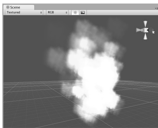
Рисунок 2. Система частиц
