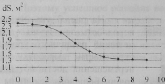
Рис. 4. Изменение поперечного сечения выработки в зависимости от количества анкеров
