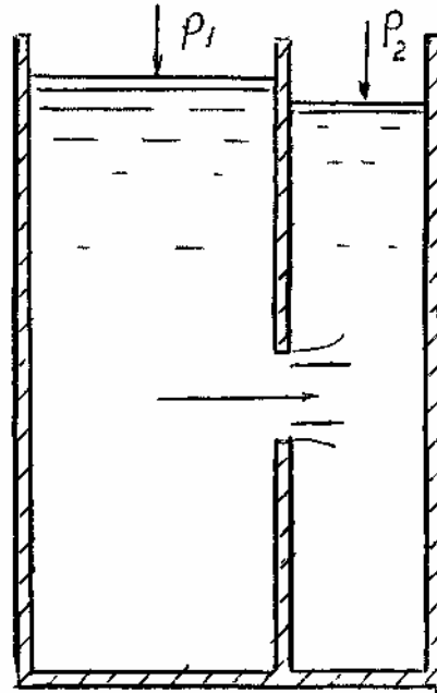
Рис. 3. Истечение жидкости из затопленного отверстия
