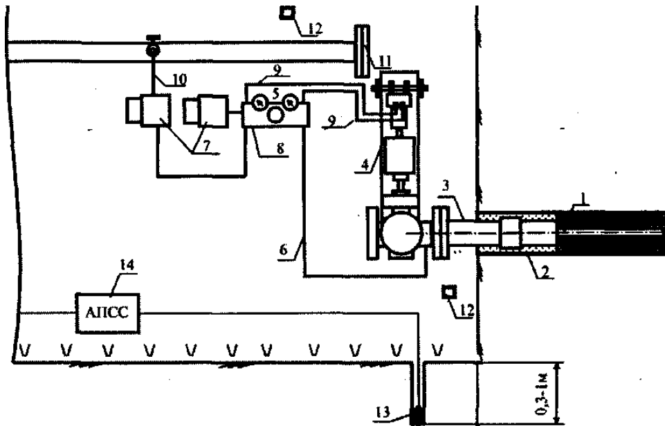
Рис. - Схема розташування обладнання для ГДД:
