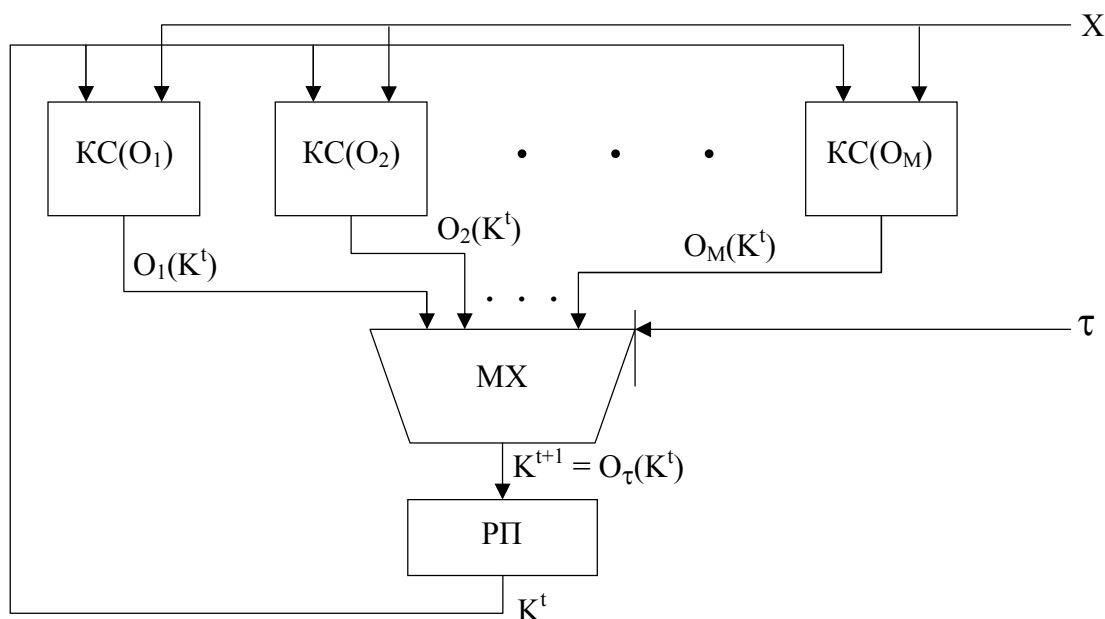
Рисунок 2 – Структурная модель ОАП с операционной частью I-типа
