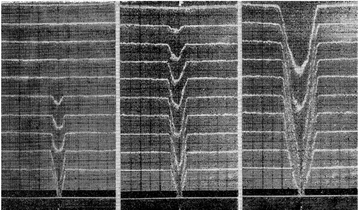
Рис.2. Стадии развития эллипсоида разрыхления в дискретной среде (Г.М. Малахов (1968)).
