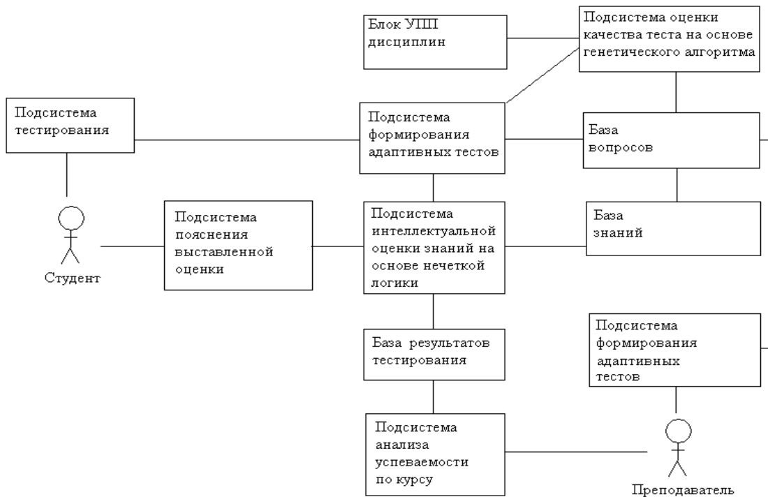
Рисунок 1 – Обобщенная структура создаваемой экспертной системы
