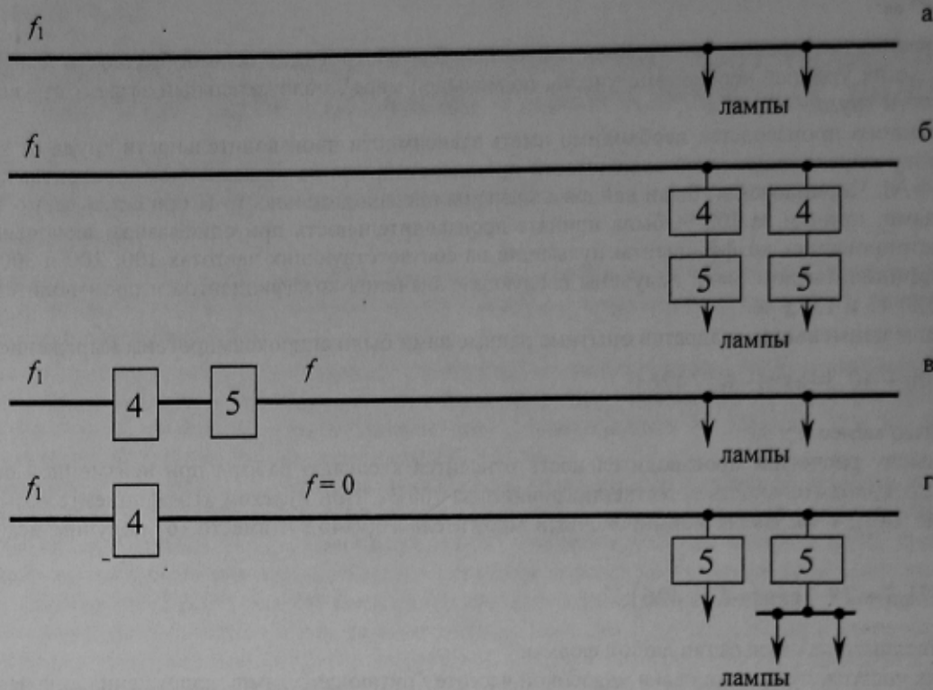
Рисунок 3 – Схемы питания ламп
