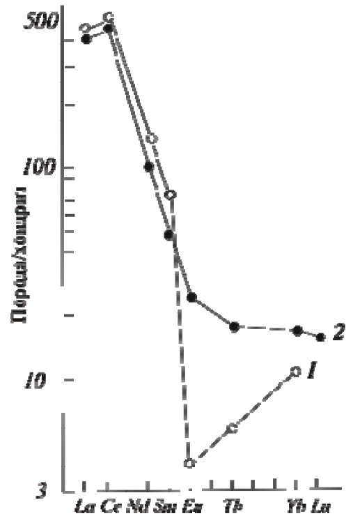
Рис. 5. Діаграма розподілу РЗЕ в салтичанських гранітах
