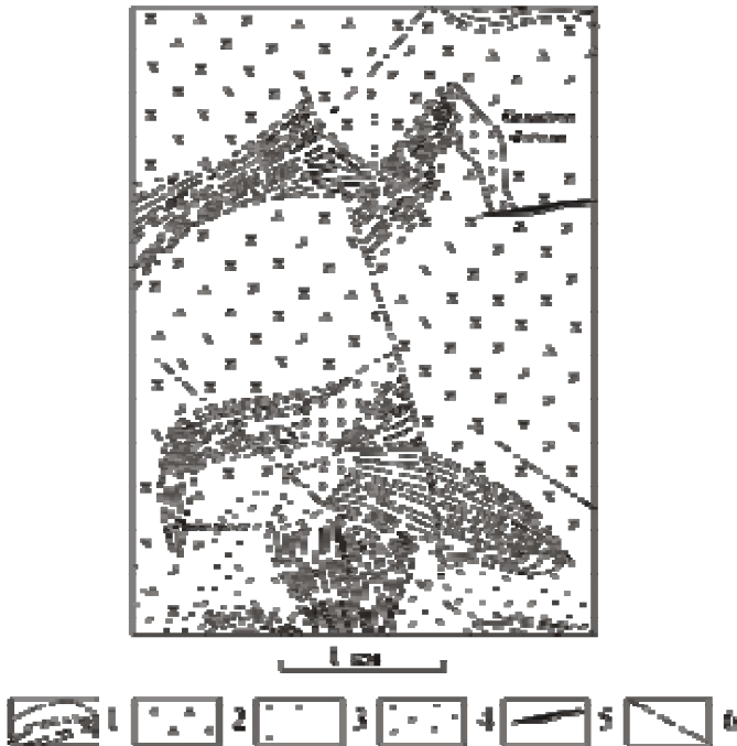
Рис. 1. Геологічна схема району с.Радолівка і Салтичої Могили
