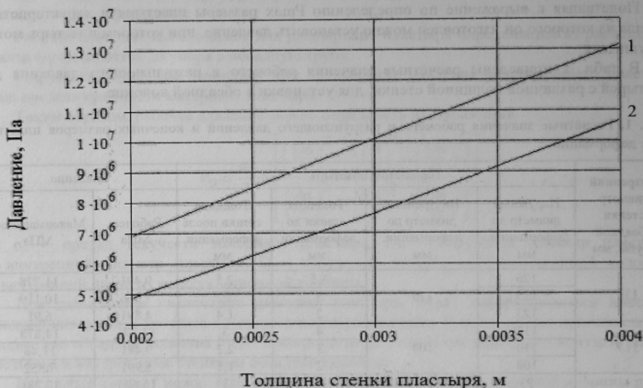
Рис. 4. Зависимость рабочего и разрушающего давлений от толщины стенки пластыря.
