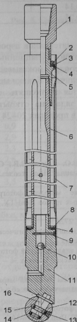
Рис. 1. Устройство установки пластырей в скважине УУП-1:
