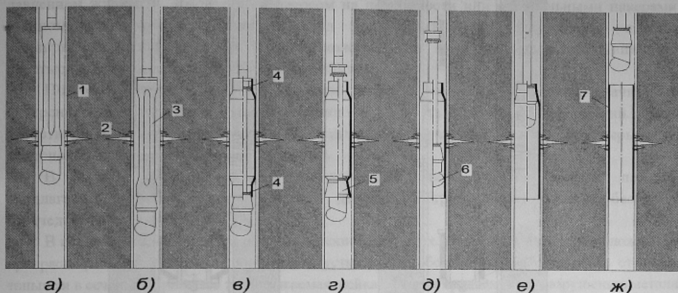
Рис. 2. Последовательность установки пластыря в обсадной колонне
