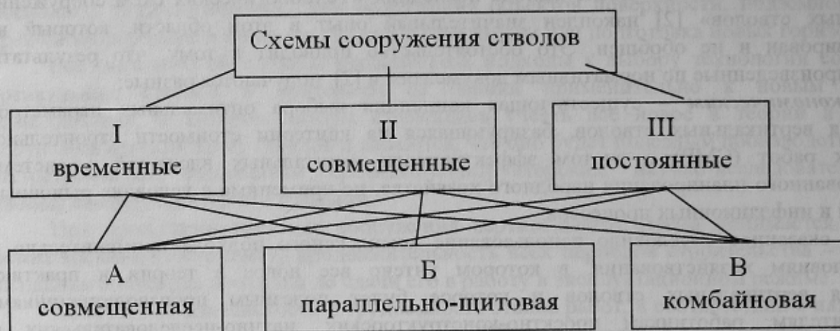
Рис.1. Классификация схем сооружения вертикальных стволов шахт
