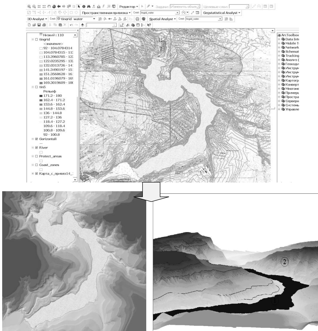
Рис. 4. Моделювання поверхневих стоків та визначення водозбірної площі для водосховища
