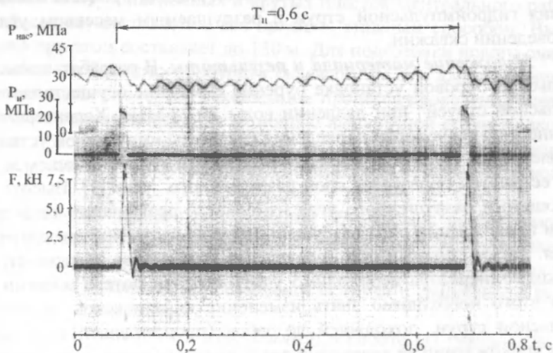
Рисунок 1 - Осциллограммы силы воздействия F и давления P_n импульсной струи при ее движении по воздуху, расстояние от насадка до преграды l = 1 м.
