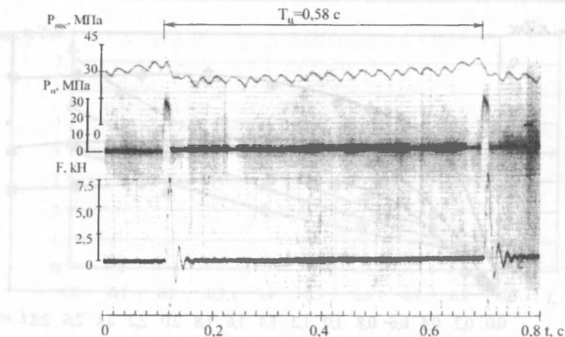
Рисунок 2 - Осциллограммы силы воздействия F и давления P_u импульсной струи при ее движении через слой разрушенного угля, толщина слоя угля L = 0,2 \text{ м} .
