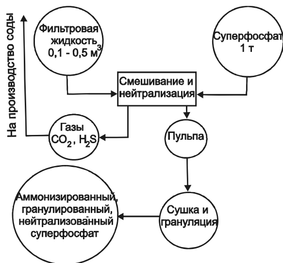
Рис. 1. Принципиальная технологическая схема переработки фильтровой жидкости содовых заводов в двойное азотно-фосфорное удобрение
