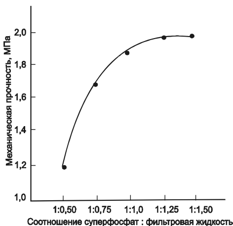
Рис.2. Влияние количества добавки фильтровой жидкости на механическую прочность гранул
