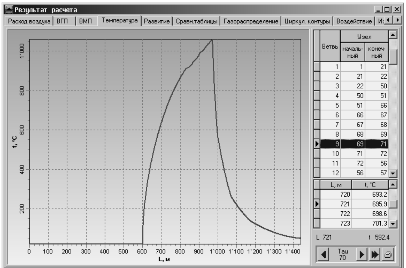
Рис.3. График температур вдоль оси выработки
