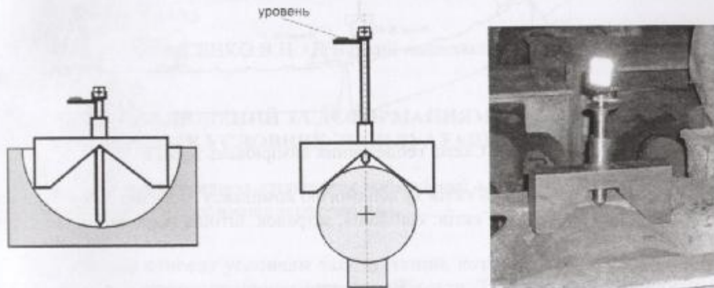
Мал.15. Вимірювання призмовою підставкою посадового гнізда підшипника (зліва) і ролику (зправа)
