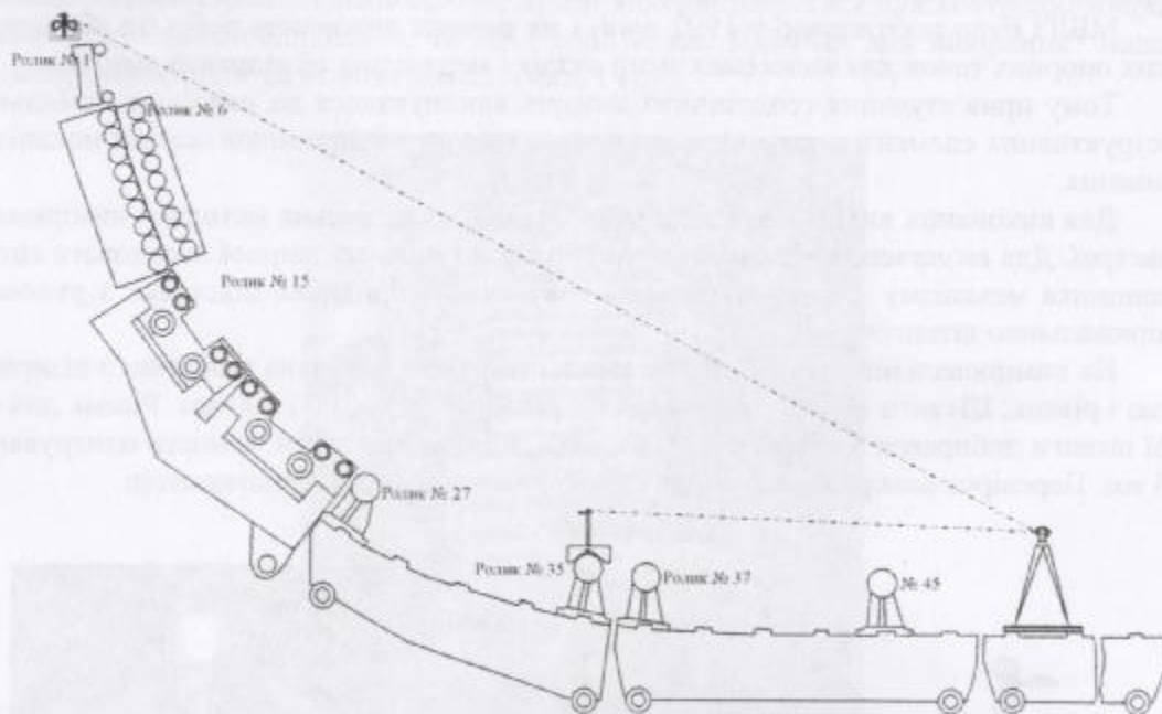
Мал. 16. Схема геодезичних вимірювань МБЛЗ
