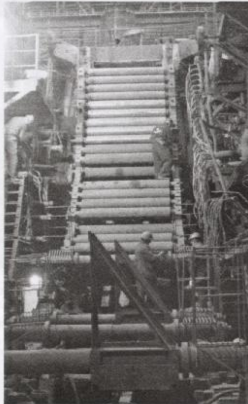
Мал. 14. Загальний вигляд МБЛЗ з встановленими шаблонами
