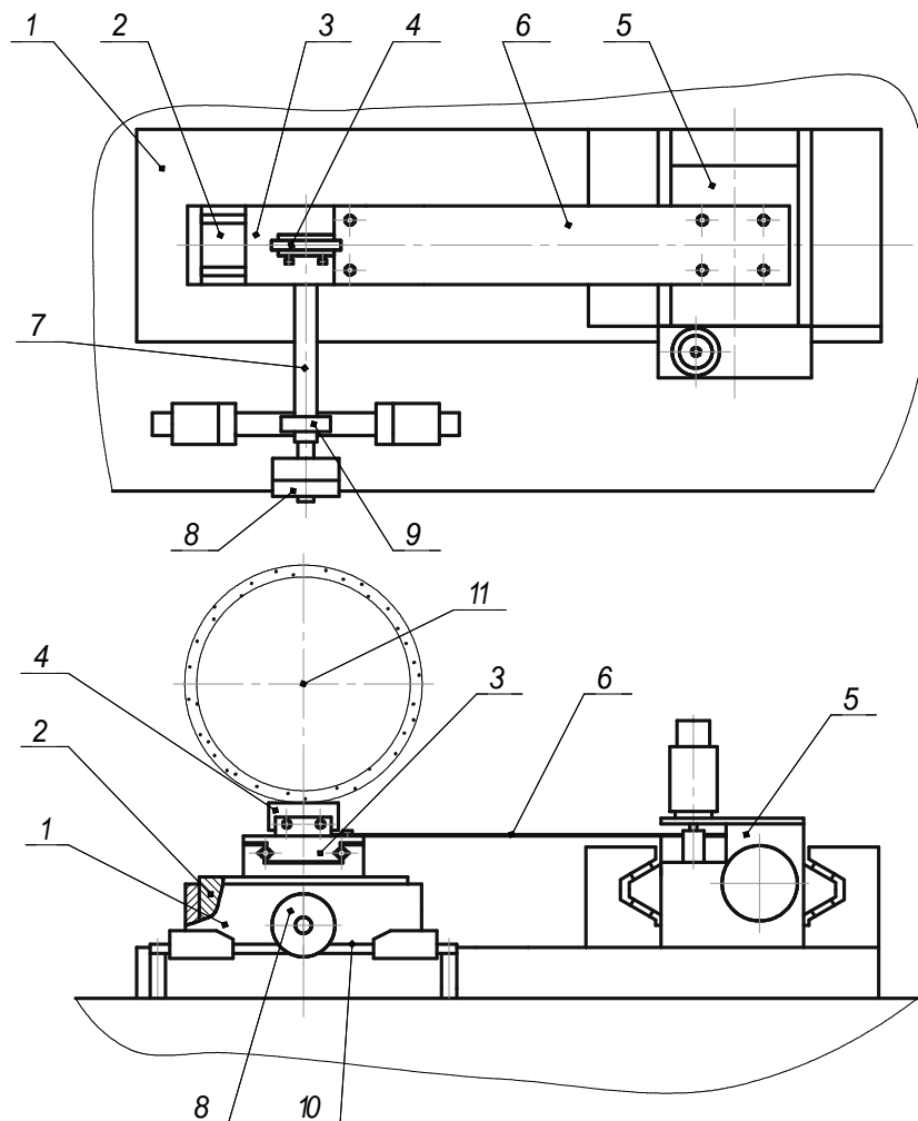
Рисунок 1 – Пристрій для шліфування за пружною схемою з накладенням вібрацій на заготовку
