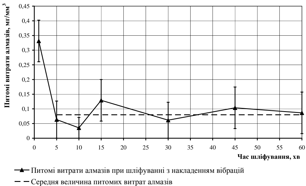
Рисунок 5 – Питомі витрати алмазів при шліфуванні сталі Р6М5Ф3 по пружній схемі без вібрацій заготовки (а) та з накладенням вібрацій
