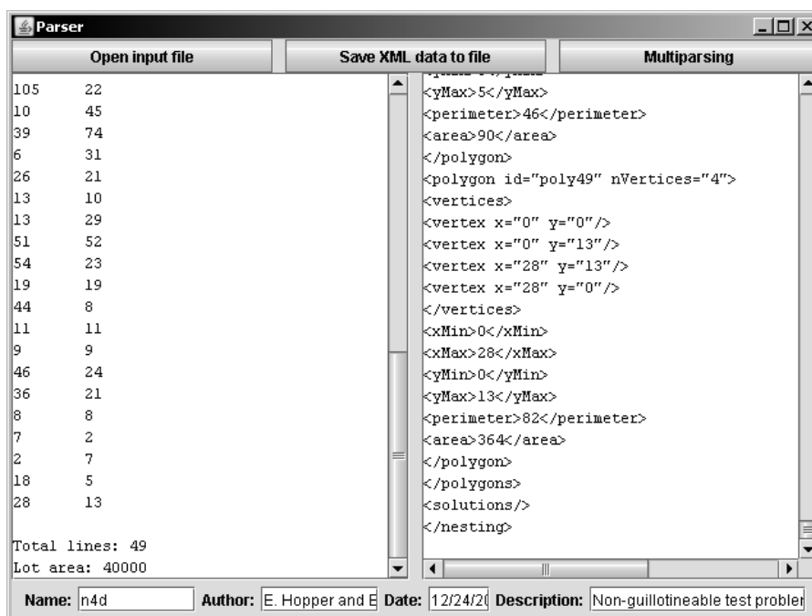
Рисунок 2 — Интерфейс парсера, реализованный с использованием средств Swing
