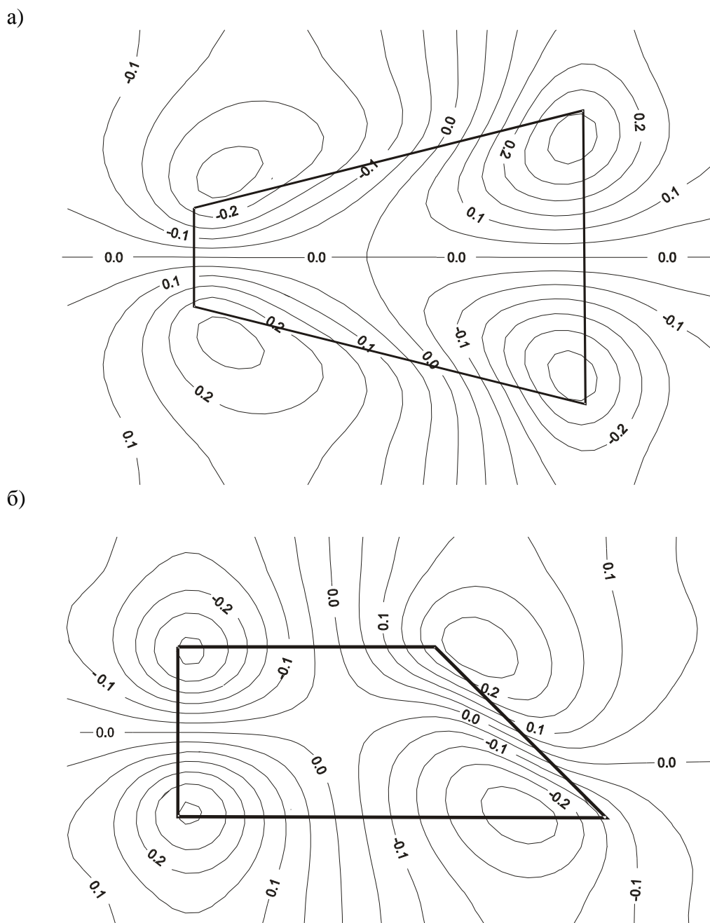
Рис. 5 Распределение деформаций скашивания вызванных выработками равномерно расширяющейся (сужающейся) (а) и клинообразной (б) формы выработок неправильной формы .
