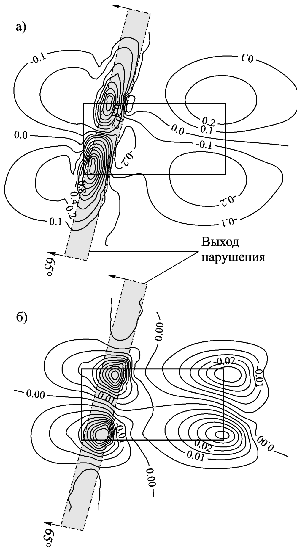
Рис. 7 Распределение деформаций скашивания (а) и скручивания (б) при подработке слабодиагонального разрыва (угол разворота от линии заборта 15^\circ )
