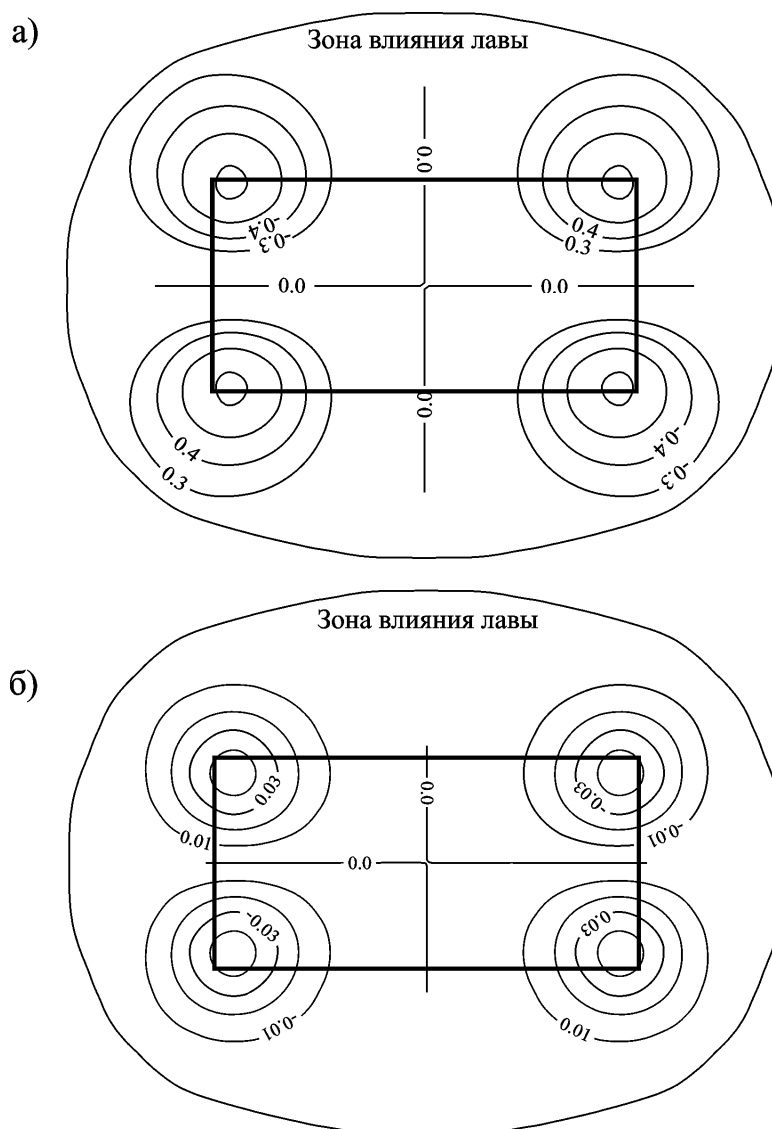
Рис. 4 Изолинии распределения деформаций скашивания (а) и скручивания (б) земной поверхности при «стандартных» условиях подработки.
