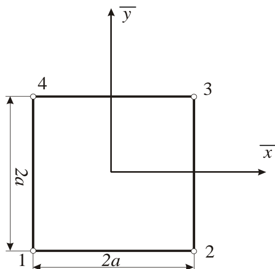
Рис. 3 Плоский четырехугольный элемент
