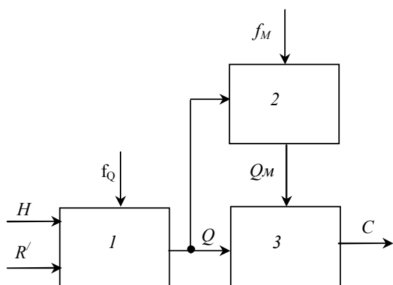
Рис. 5. Структура схемы проветривания первого типа
