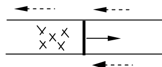
Рис.1. Тип схемы проветривания 2-В-Н-в-вт [2].
