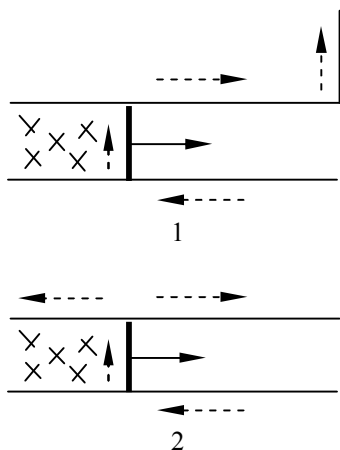
Рис.2. Типы схем проветривания: 1 - 1-М-Н-в-вт (первый период); 2 - 1-К-Н-в-вт [2].
