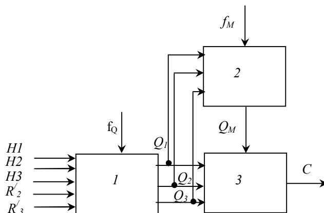
Рис. 6. Структура схемы проветривания второго типа
