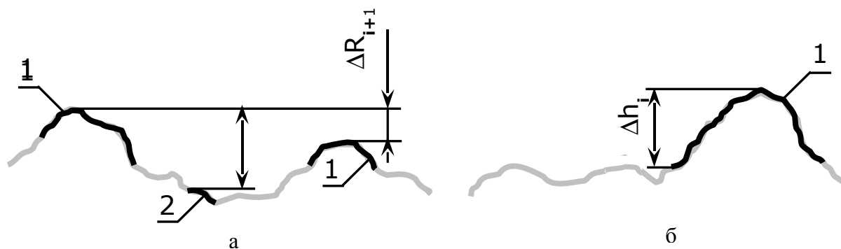
Рис. 4. Определение параметров рабочей поверхности круга: а – разновысотности зерен; б – выступления зерен из связки
