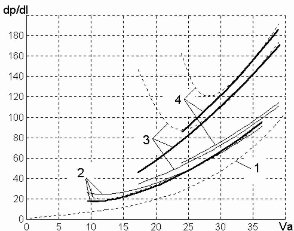
Рис.2. Удельные потери давления при транспортировке солода и золы
