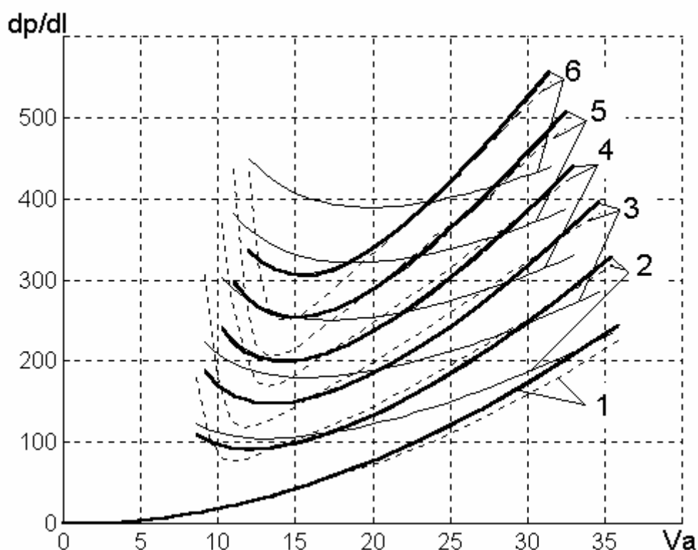
Рис.1. Удельные потери давления в трубопроводе при транспортировке полистирола
