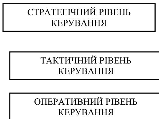
Рис. 1.3 – Рівні керування
