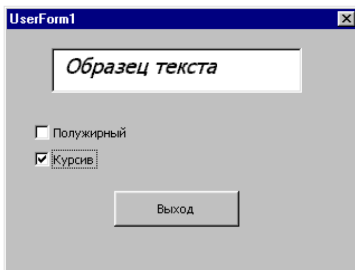
Рис. 10.10 - Використання прапорців
