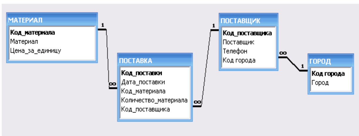
Рис. 9.1 – Схема даних
