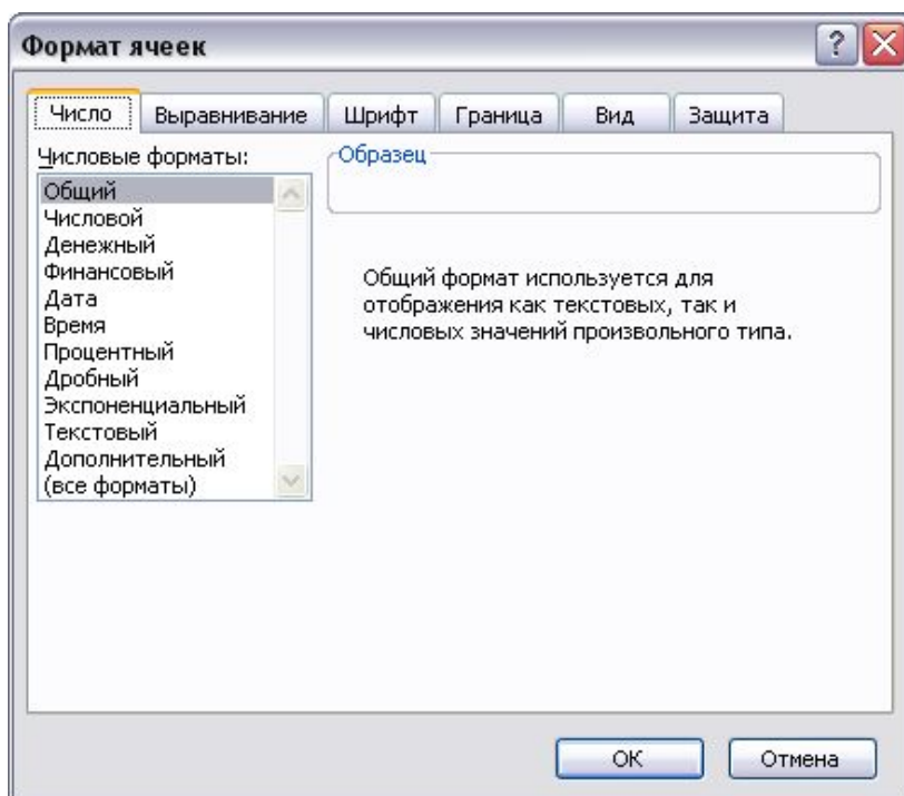
Рис. 8.23 – Вкладка "ЧИСЛО"
