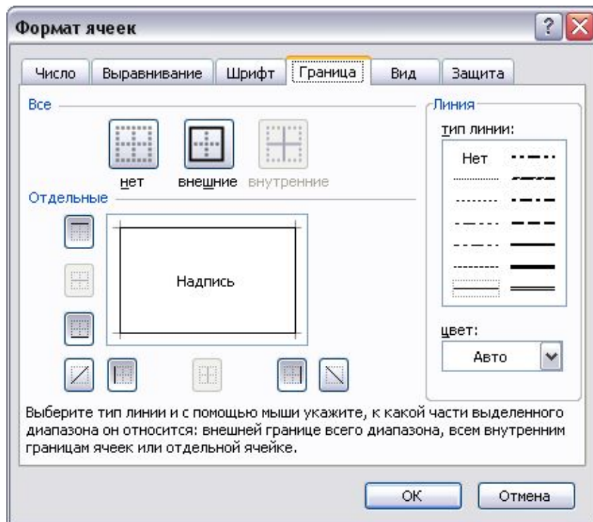
Рис. 8.26 – Вкладка "ГРАНИЦА"
