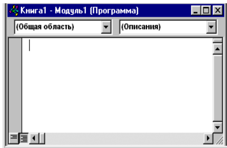
Рис. 10.5 - Вікно модуля
