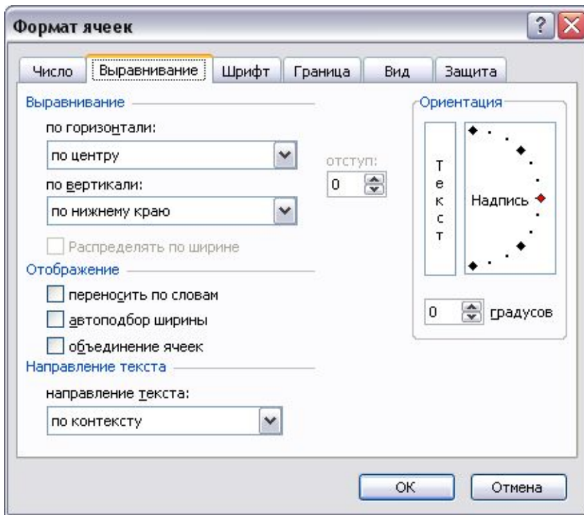
Рис. 8.24 – Вкладка "ВЫРАВНИВАНИЕ"
