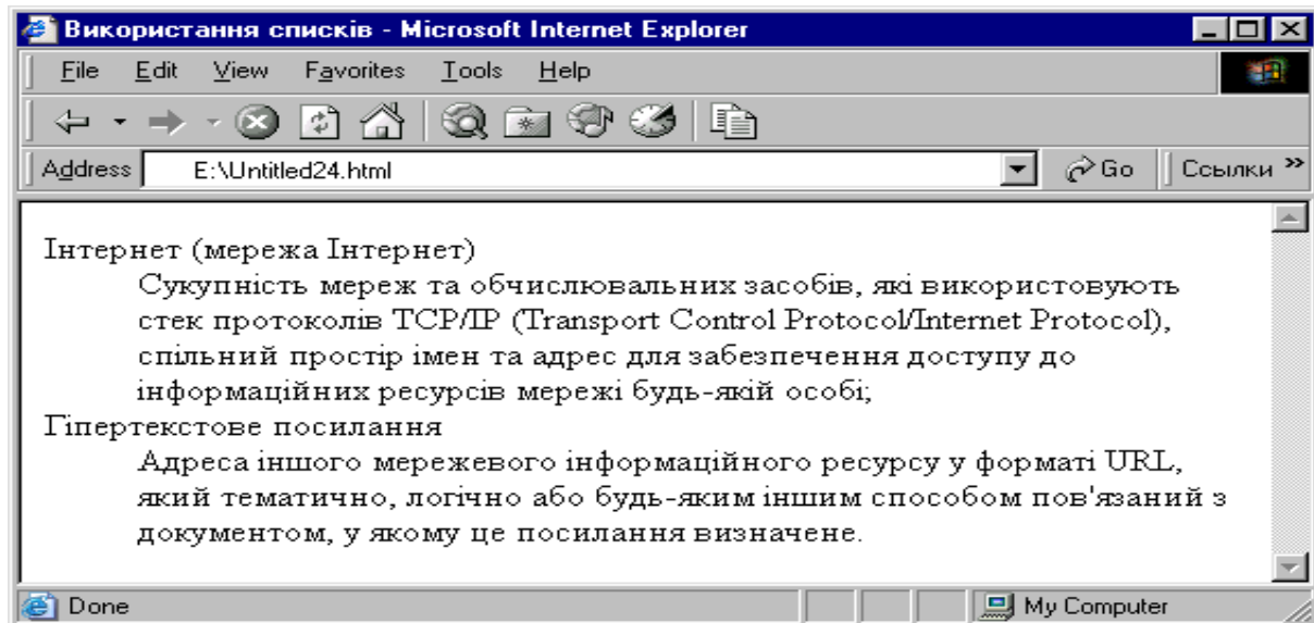
Рис. 7.11 - Список визначень
