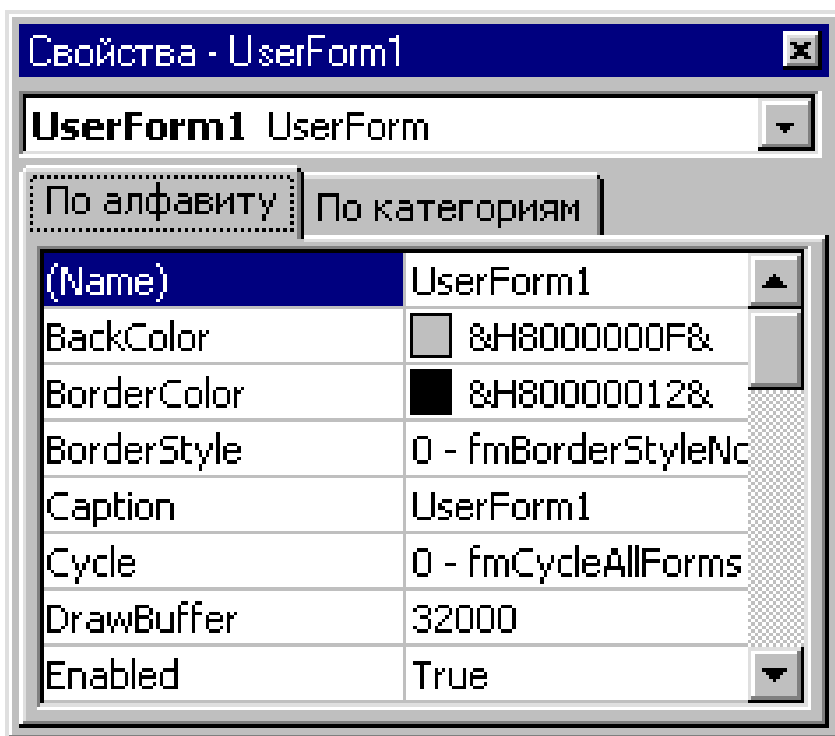
Рис. 10.4 - Вікно властивостей
