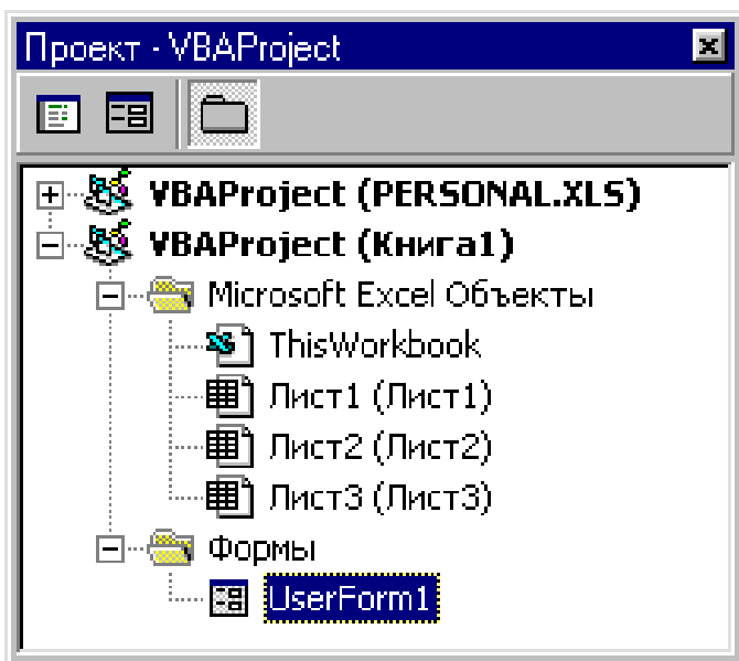
Рис. 10.3 - Вікно проекту
