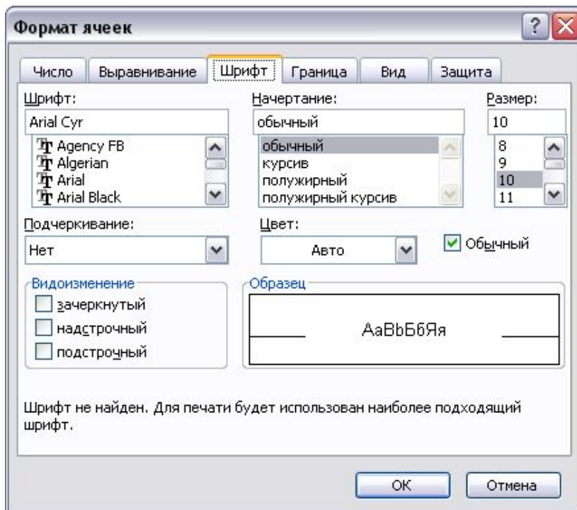
Рис. 8.25 – Вкладка "ШРИФТ"
