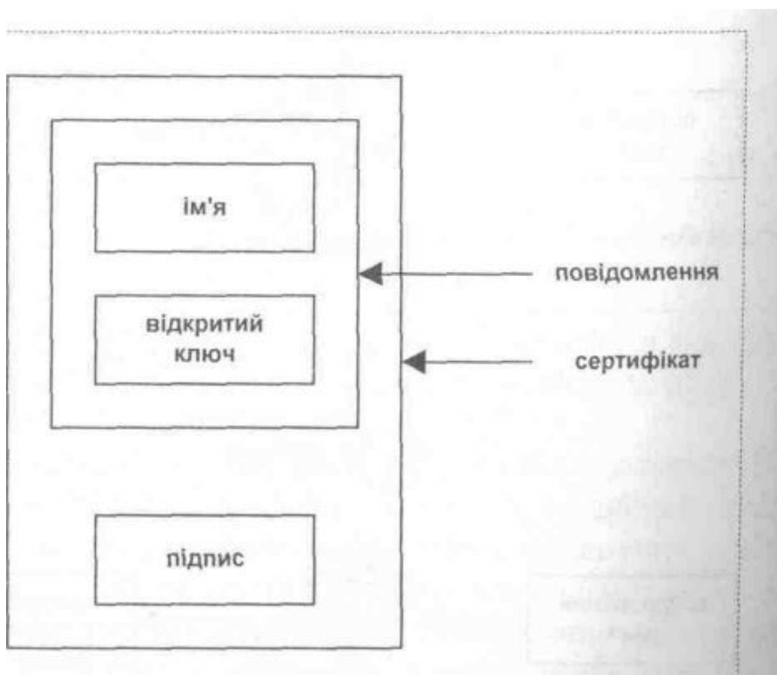
Рис. 6.4 - Цифровий сертифікат
