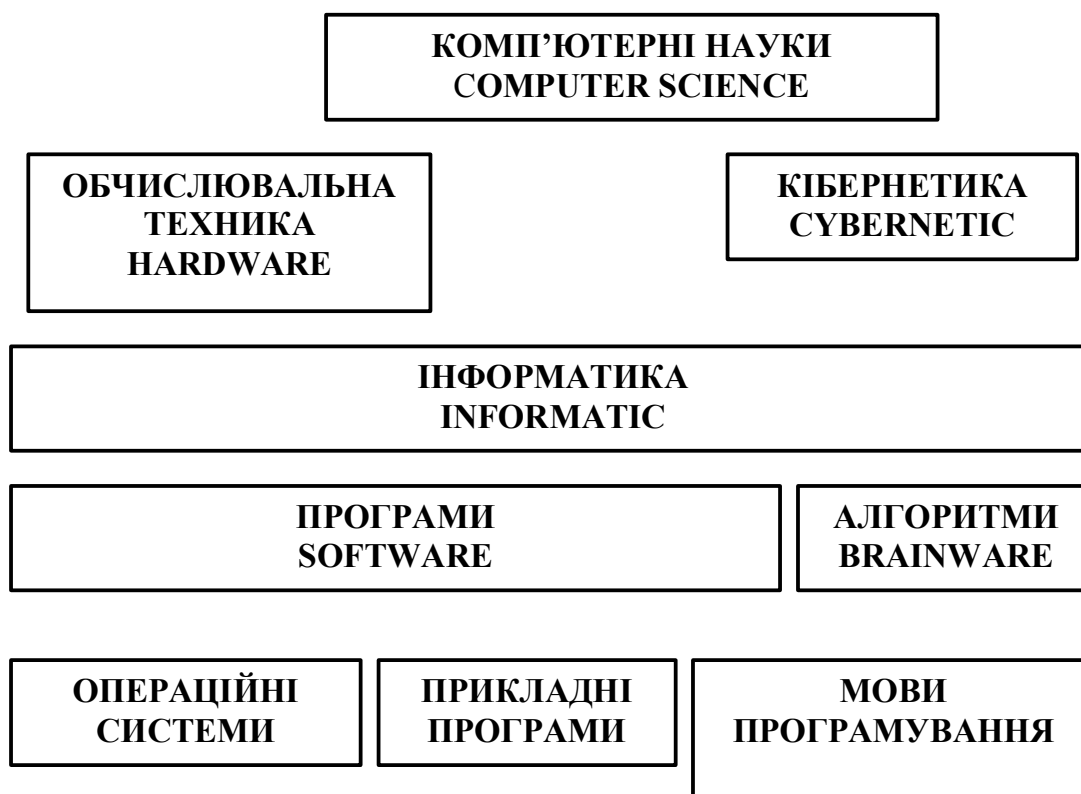
Рис. 1.1 - Структура інформатики
