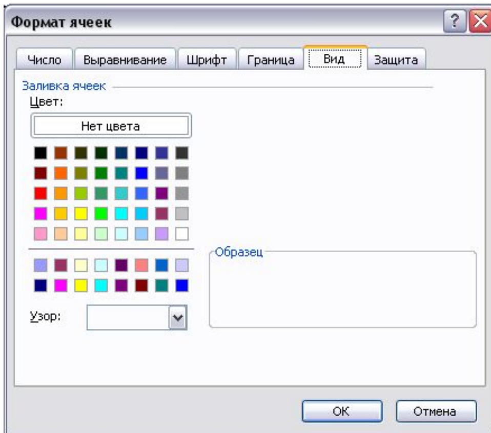
Рис. 8.27 – Вкладка "ВИД"
