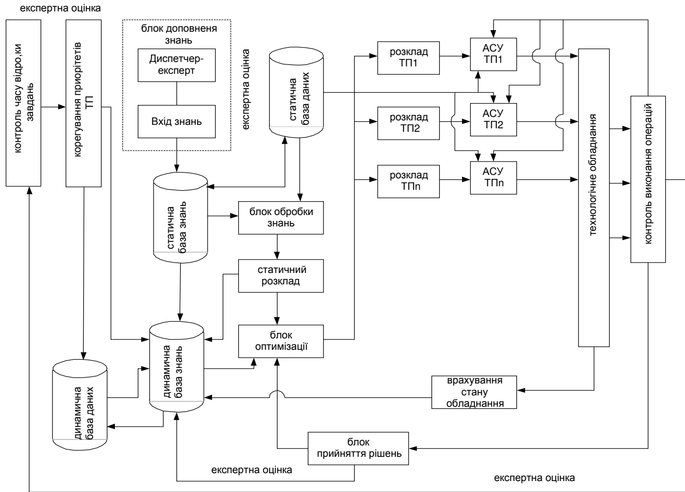
Рис. 2. Функціональна схема формування оптимального розкладу управління технологічними лініями з використанням експертних оцінок
