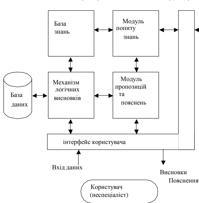
Рис. 1. Базова структура експертної системи
