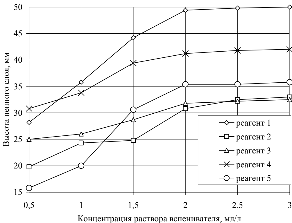
Рис. 2 – Зависимость высоты пены от концентрации реагентов
