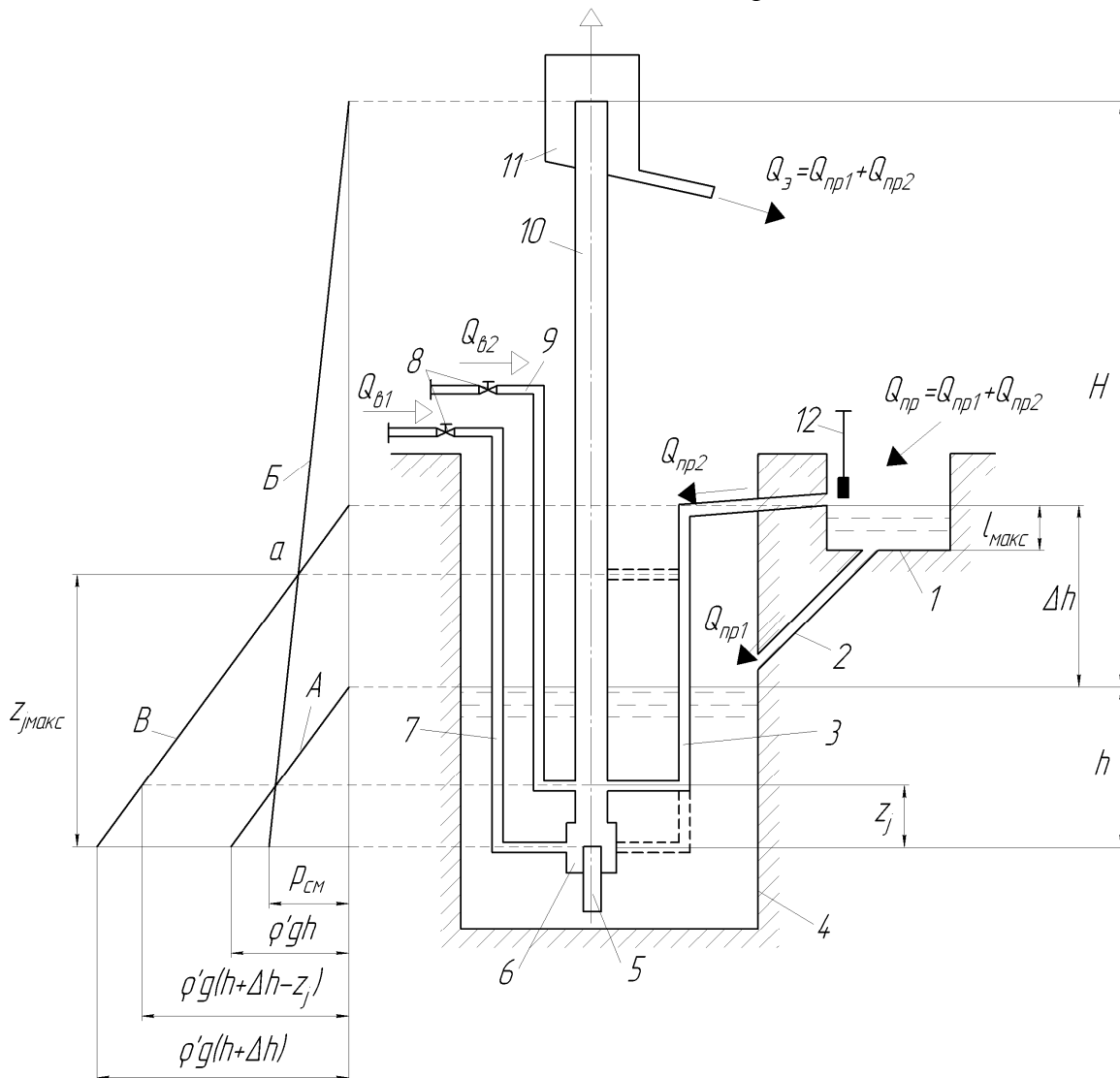
Рисунок 1 - Схема эрлифтной установки с подводом дополнительного притока жидкости (гидросмеси) в промежуточное сечение подъемной трубы: 1 - приемная емкость; 2 - основной подводный трубопровод; 3 - дополнительный подводный трубопровод; 4 - зумпф; 5 - подающая труба; 6 - смеситель; 7 - основной воздухопровод; 8 - задвижки; 9 - дополнительный воздухопровод; 10 - подъемная труба; 11 - воздухоотделитель; 12 - запорное устройство; A - эпюра давления жидкости (гидросмеси) в зумпфе 4; B - эпюра давления газожидкостной смеси (аэрогидросмеси) в подъемной трубе 10; B - эпюра давления жидкости (гидросмеси) в дополнительном подводном трубопроводе 3
