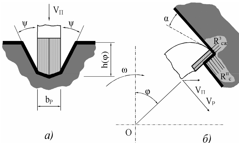
Рисунок 2 – Характер напряженного состояния угля разрушаемого массива
