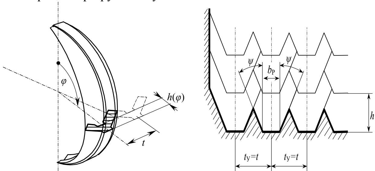
Рисунок 1 – Характер «вырезаемой» резцами части пласта а) и характер его разрушения б) при последовательном резе
