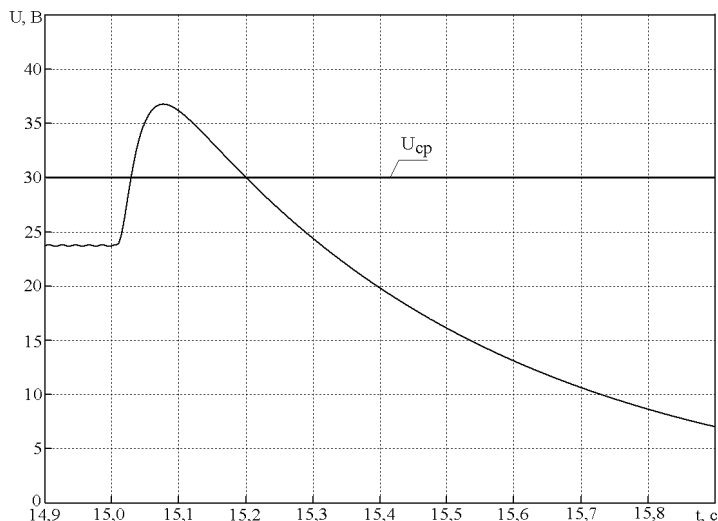
Рисунок 2 - Діаграма напруги на вимірювальному елементі апарату захисту від витоку струму на землю при відключенні відгалуження
