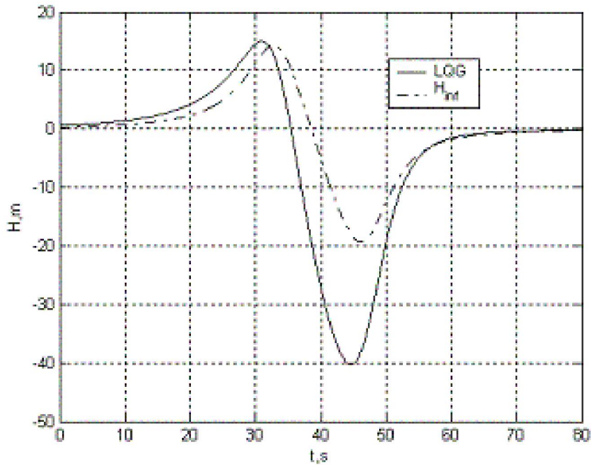
Рисунок 2 – График отклонения высоты H при использовании ЛКГ и H^\infty – субоптимального регулятора
