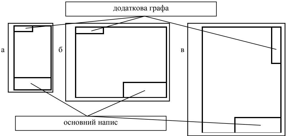
Рисунок 4.1. Розташування основних написів у студентських роботах: а) для формату А4; б) для форматів більше А4 при розташуванні основного напису уздовж довгої сторони аркуша; в) для форматів більше А4 при розташуванні основного напису уздовж короткої сторони аркуша
