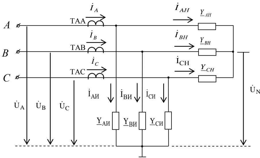
Рисунок 2 - Схема замещения присоединения нагрузки в сети с изолированной нейтралью
