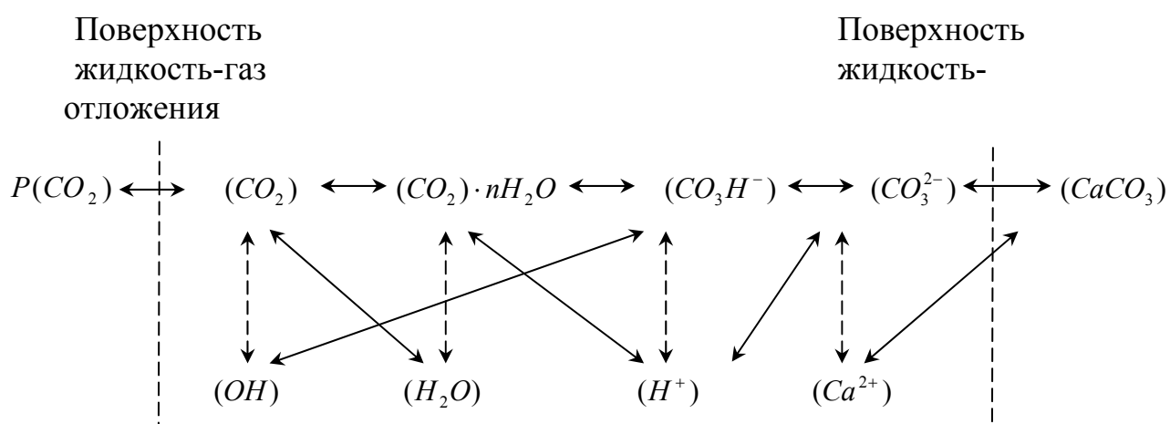
Рис. 1. Диаграмма равновесия разных модификаций карбоната кальция
